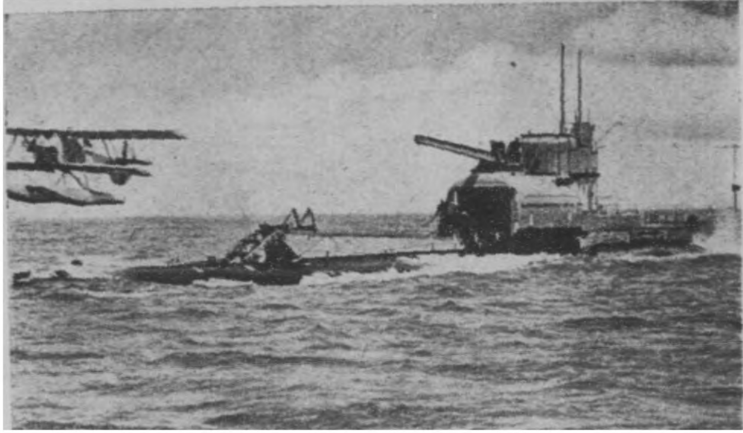
英國潛水艇。艇上可收容飛機
