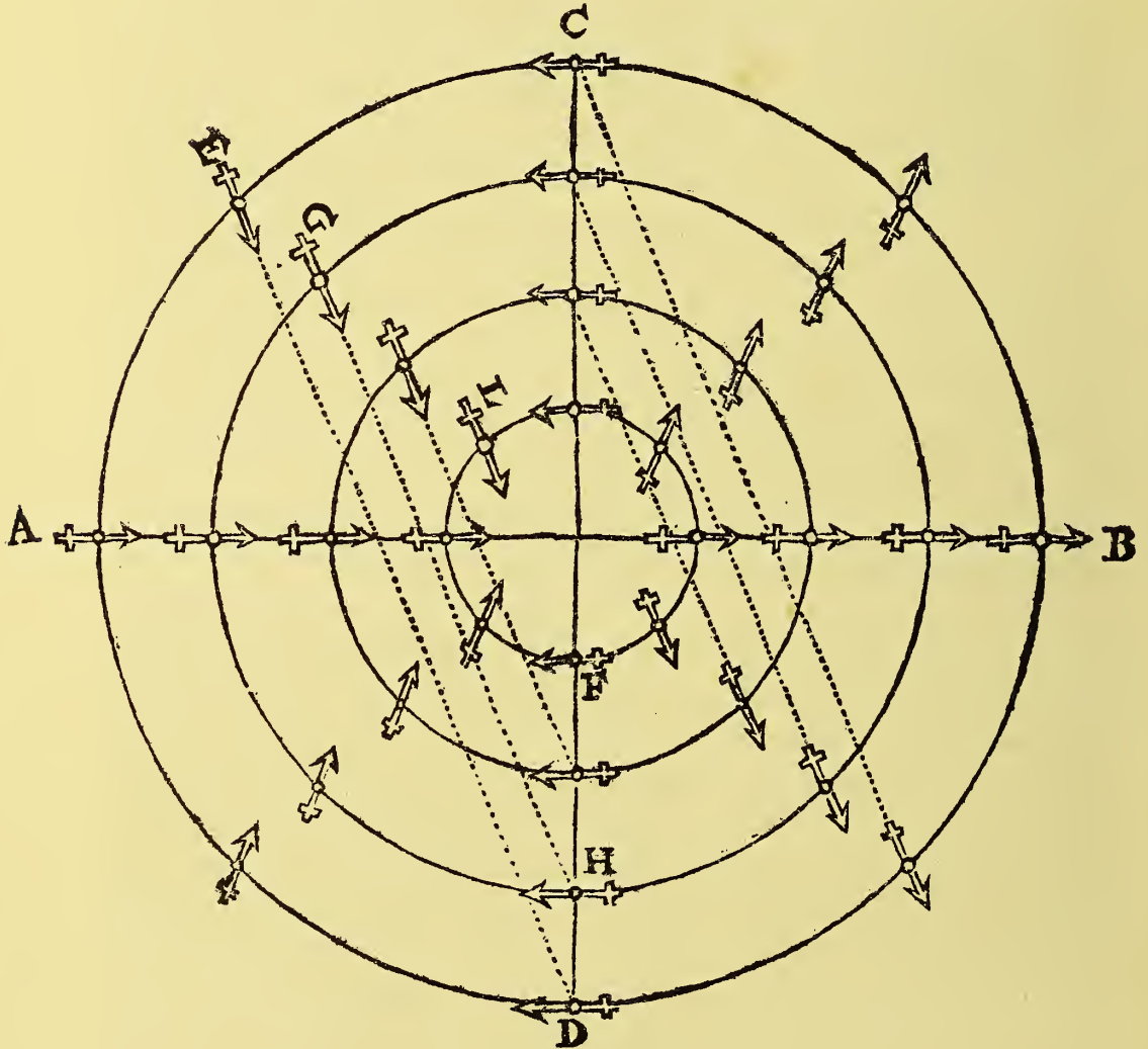
Diagramma motuum in orbibus magneticis.
