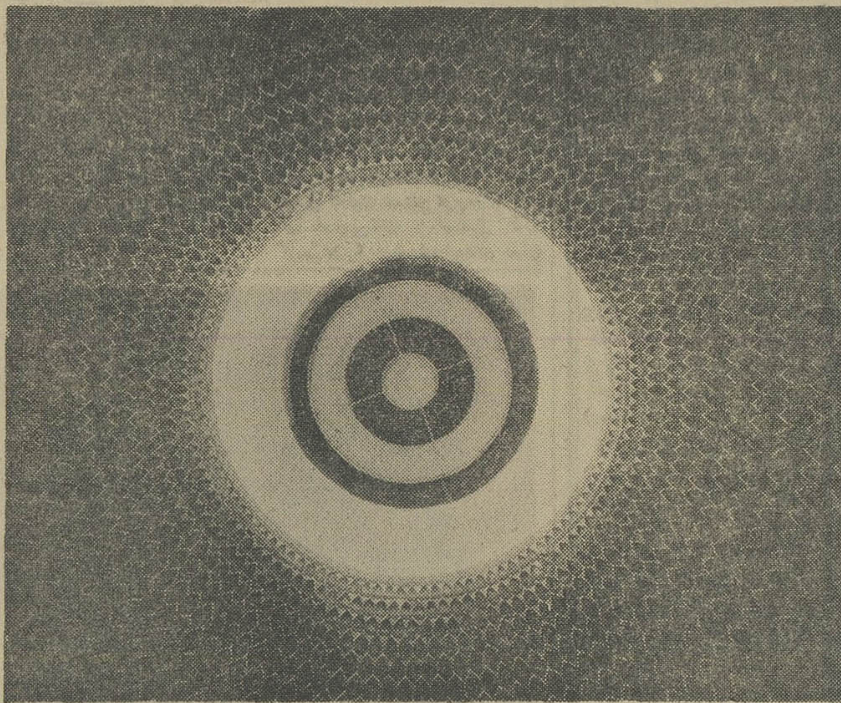
سقف مشبك فلزی سالن ولوستر مدور وسط سالن که ۷ متر قطر آن است . در وسط این لوستر نورافکن های صحنه نصب شده است
