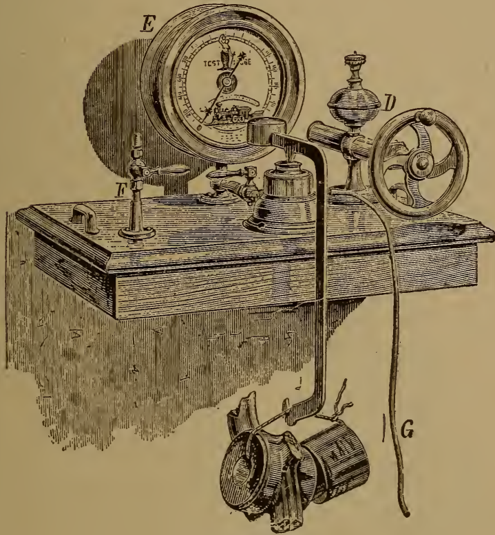
FIG. 41. Utica Gauge Tester.
