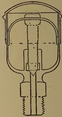
Fig. 2. Guide Cup.
