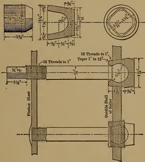
FIG. 1. Johnstone Flexible Stay Bolt.
