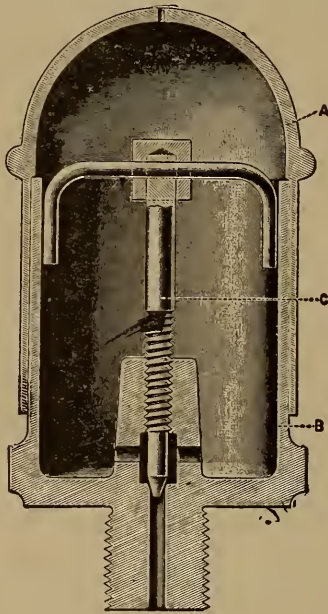
FIG. 1. Guide Cup.
