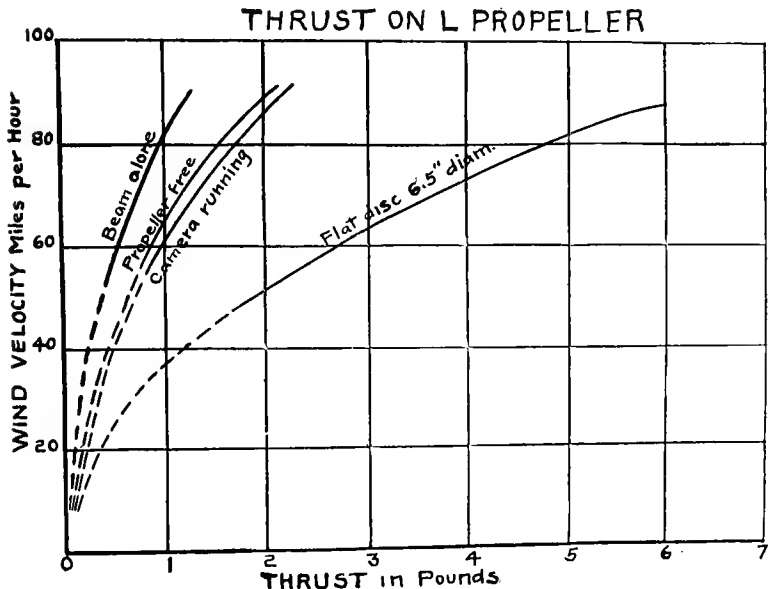
FIG. 66.—Wind propeller data.
