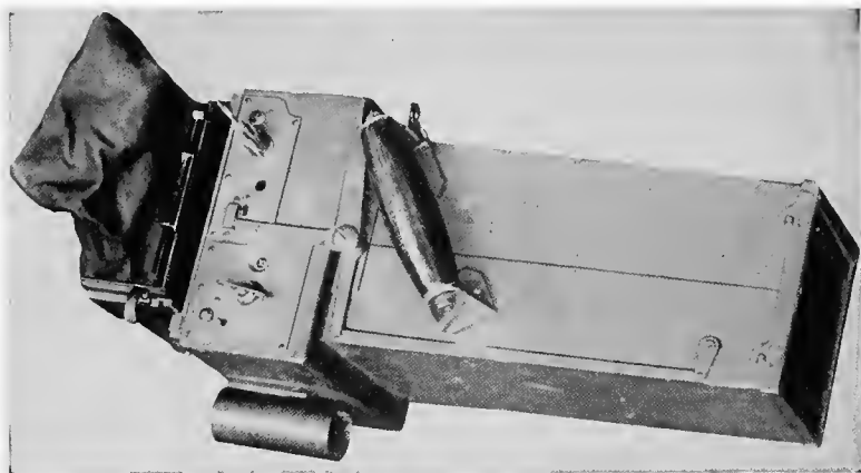
FIG. 31.—Aerial hand camera (U. S. type A-2).
