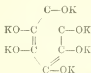
Hexaoxybenzene-potassium.
