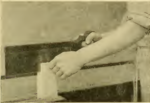
2. Finishing a Tenon.
