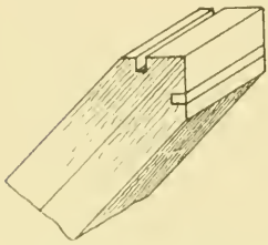
1. Tongueing a Mitre.
