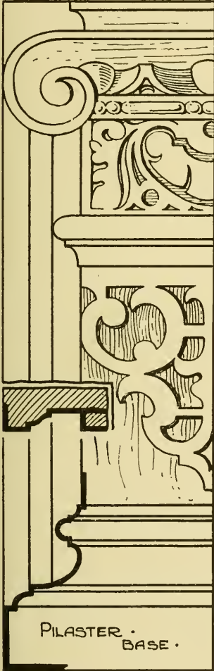
DETAIL · OF · PILAS · TER · CAP · STRAP · WORK · AND · BASE
