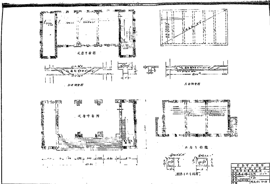
大門樓各層平面圖
