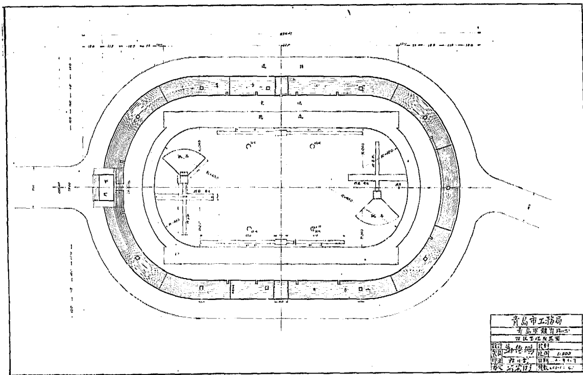
田徑賽場配置圖
