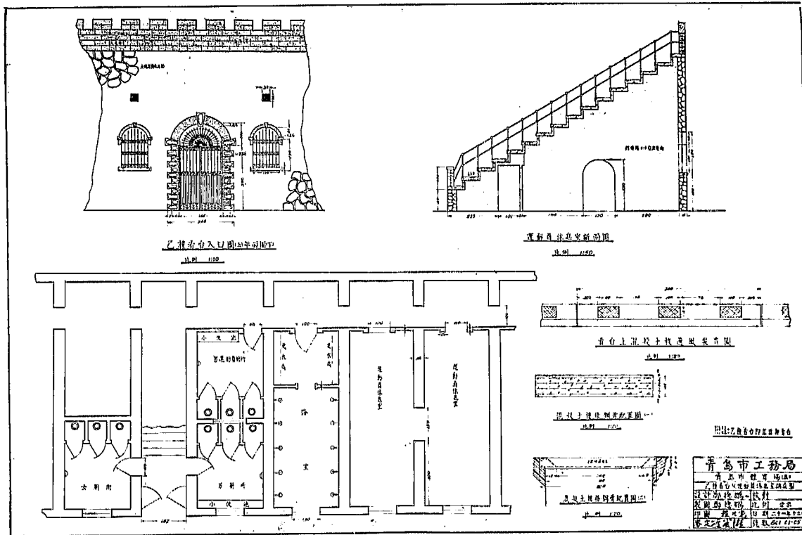
7. 乙種看台及運動員休息室構造圖
