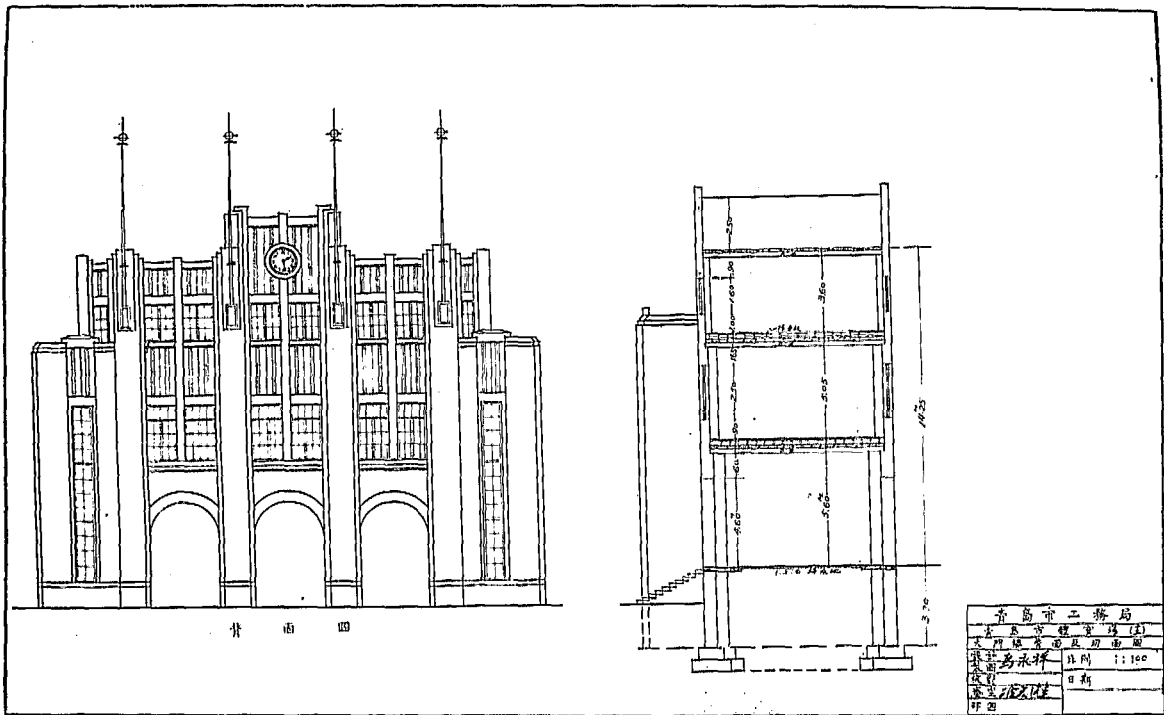
大 門 樓 背 面 及 切 面 圖
