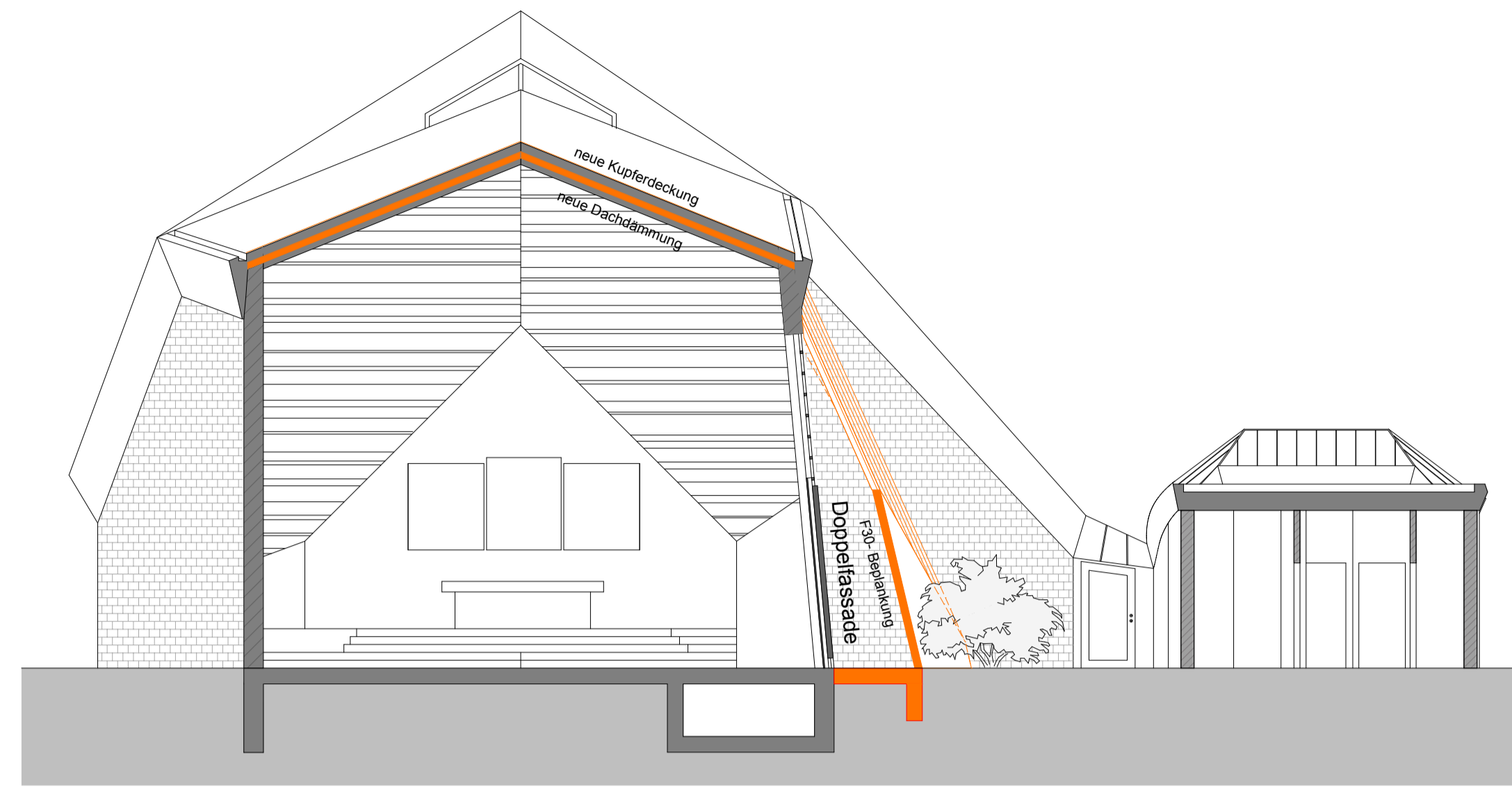
Querschnitt
