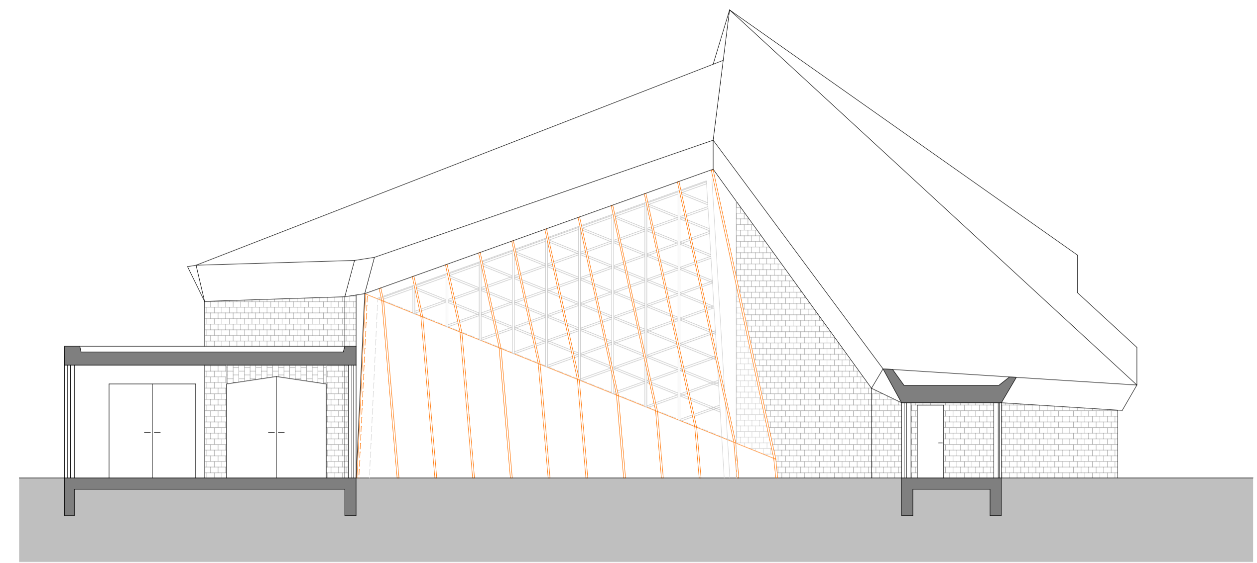
Längsschnitt mit Ansicht vom Hof
