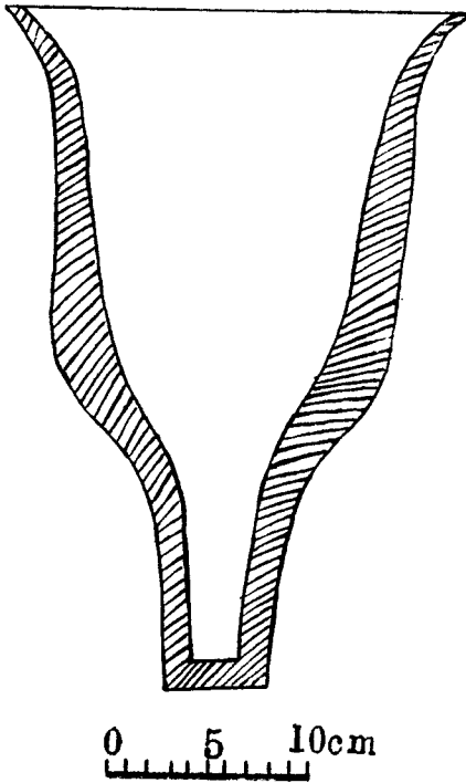
將軍盔（煉鍋）的豎剖面
