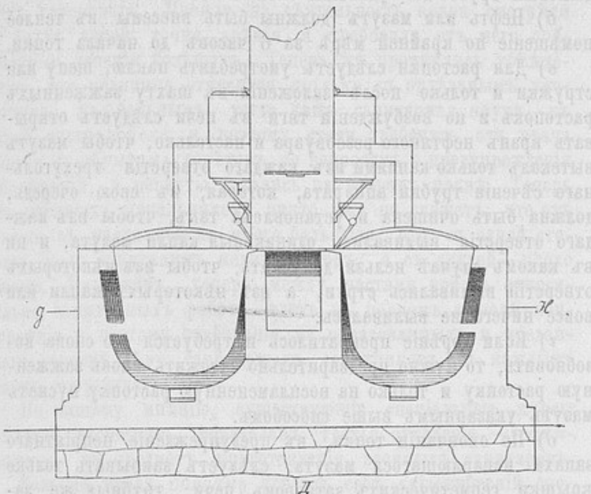
Котлы для варки пищи и нагрѣва воды для нефтяного отопленія по проекту Е. В. Мельницкаго съ трубкою капельницею инженера Кузьмина. Разрѣзь по А В.
