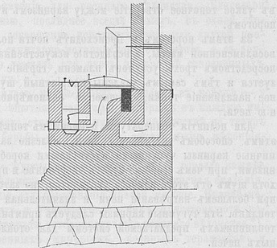
Котлы для варки пищи и нагрѣва воды для нефтяного отопленія по проекту Е. В. Мельницкаго съ трубкою капельницею инженера Кузьмина. Разрѣзь по С Д.
