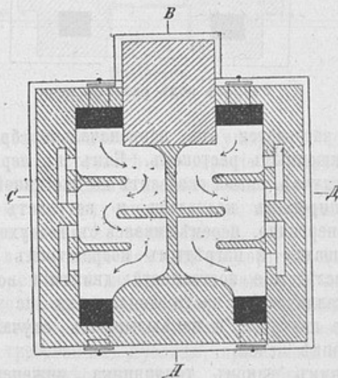
Разрѣзь по дымоходамъ подъ подомъ.
