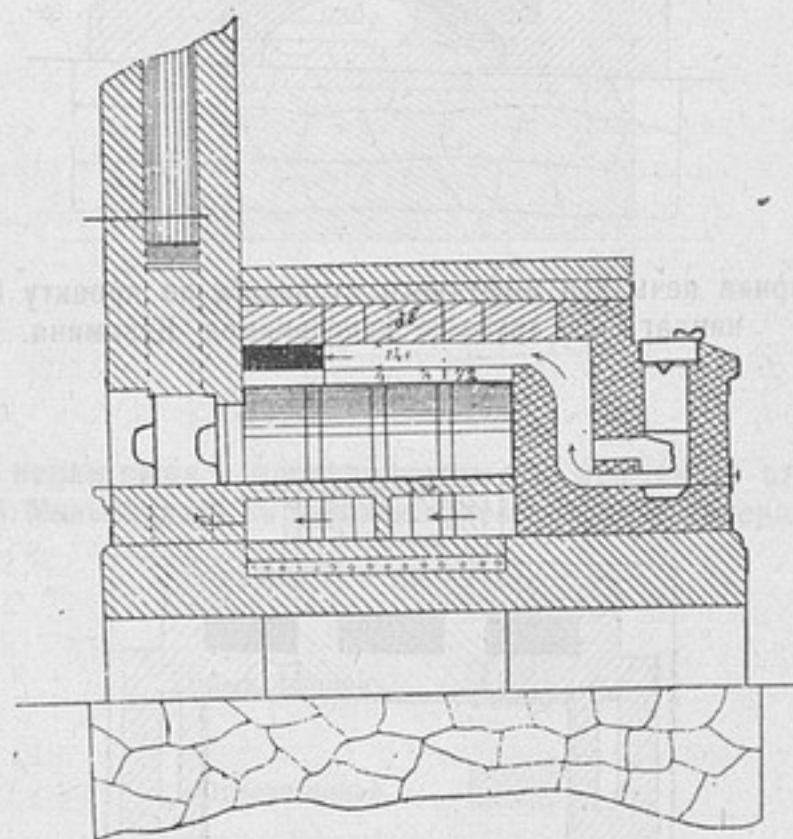
Хлѣбопекарная печь для нефтяного отопленія по проекту Е. В. Мельницкаго съ трубною капельницею Кузьмина.
