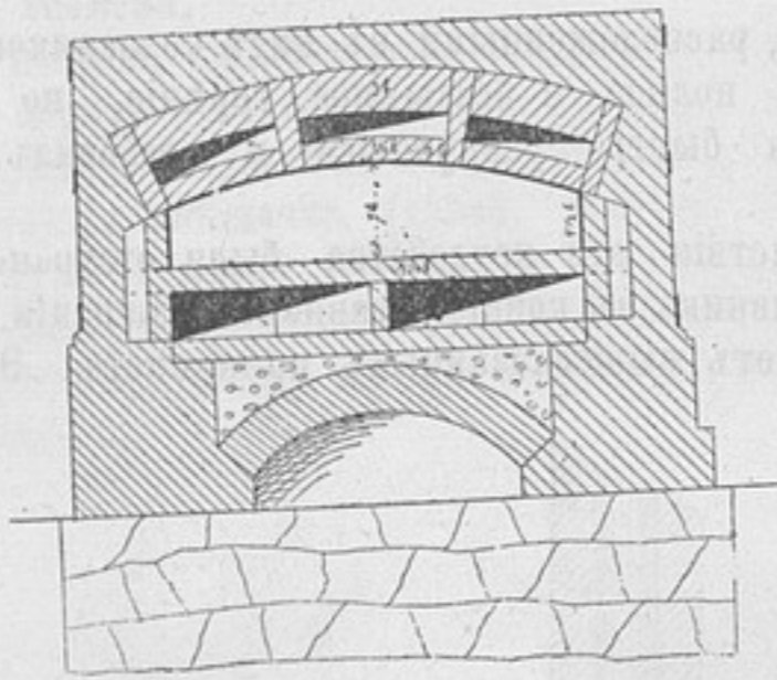
Хлѣбопечарная печь для нефтяного отопленія по проекту Е. В. Мельническаго съ трубкою капельницею Кузьмина.
