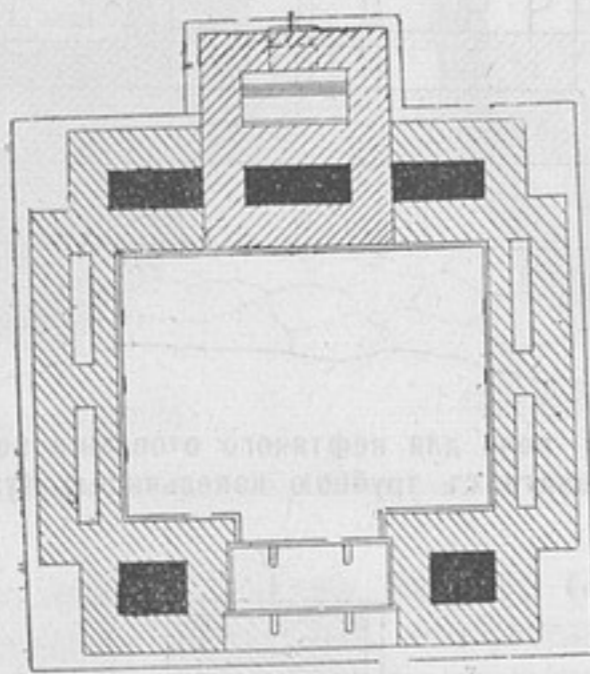
Разрѣзь подъ сводомъ печи.
