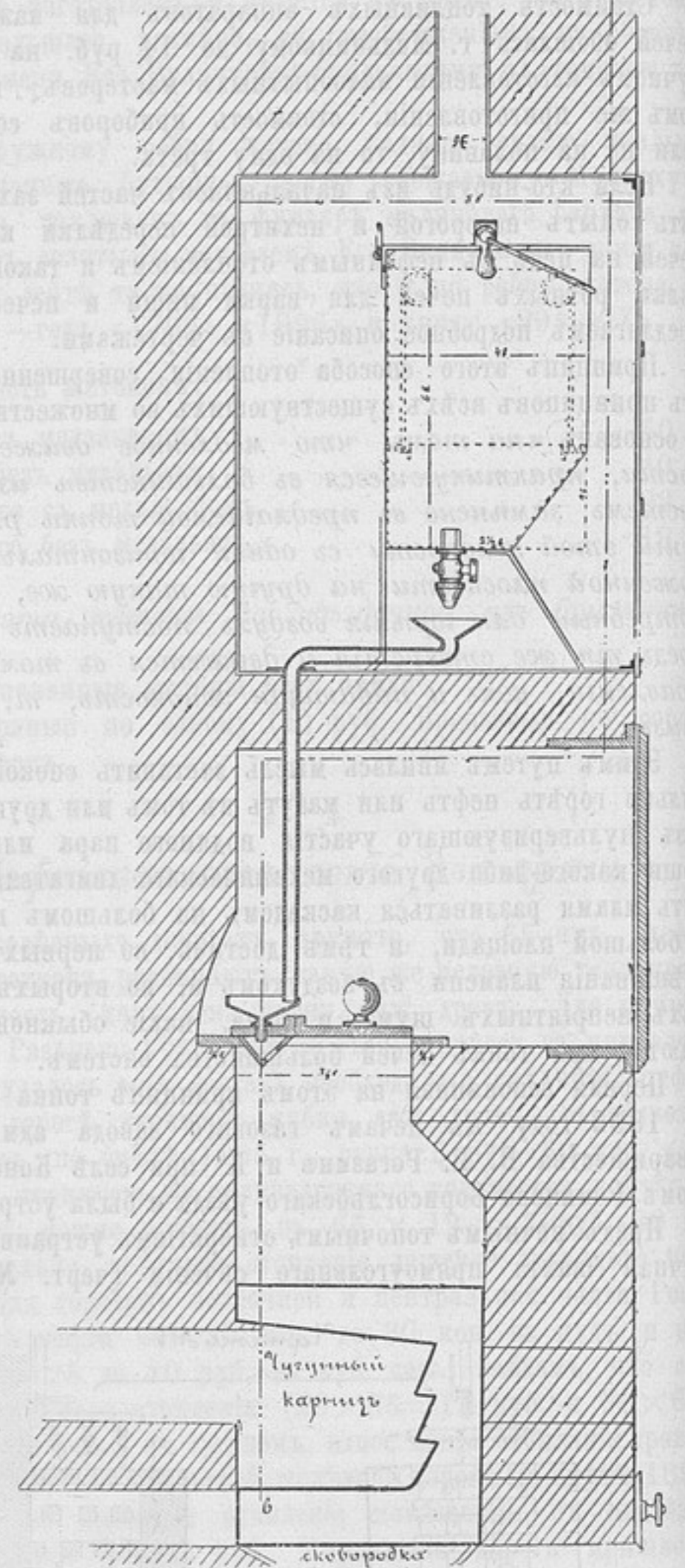
Хлѣбопечарная печь для нефтяного отопленія по проекту Е. В. Мельническаго съ трубкою капельницею Кузьмина.
