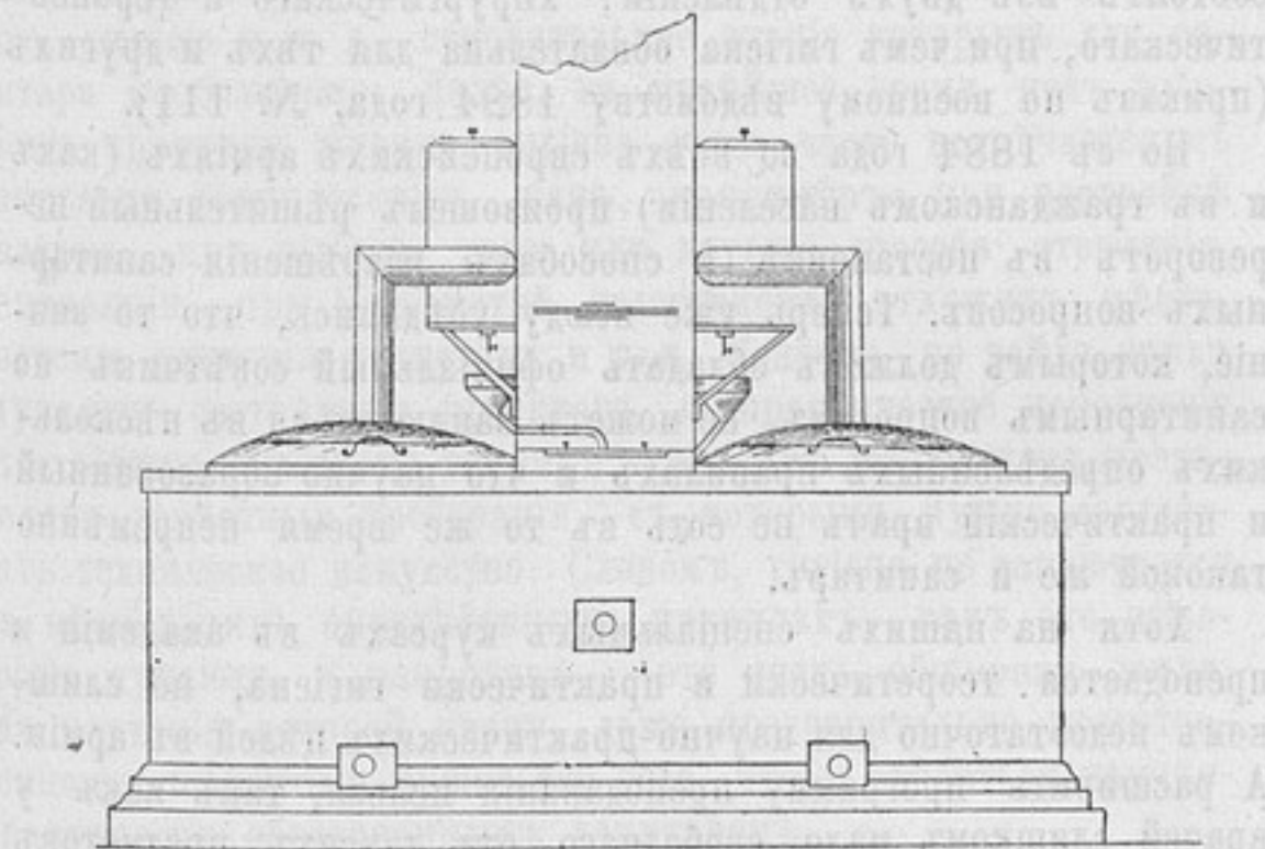
Котлы для варки пищи и нагрѣва воды для нефтяного отопленія по проекту Е. В. Мельницкаго съ трубкою капельницею инженера Кузьмина. Передній видъ.
