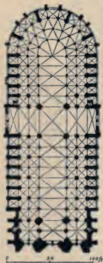
FIG. 116.—PLAN OF NOTRE DAME, PARIS.
