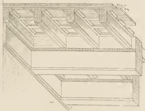
Fig. 63. Decke im Erdgeschoss des Hoetel Madrid in Sevilla.
