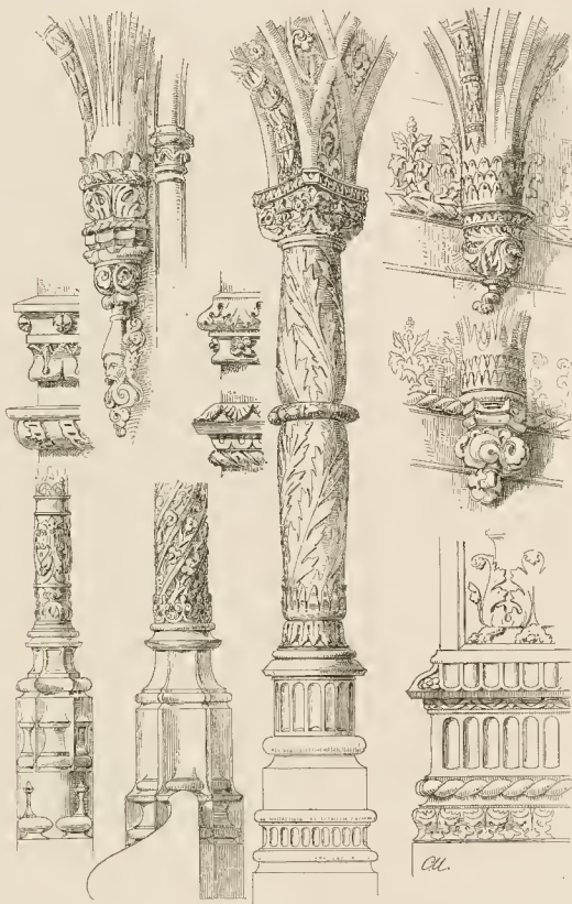
Fig. 139. Einzelformen aus dem Kreuzgang St. Jeronimus zu Belem bei Lissabon, erbaut 1517—1550.
