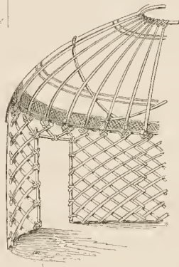
Fig. 67. Lattengeruest eines Kirgisenzeltes.
