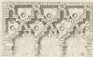
Fig. 50. Von der Cathedrale (Acusserza) in Zaragoza.
