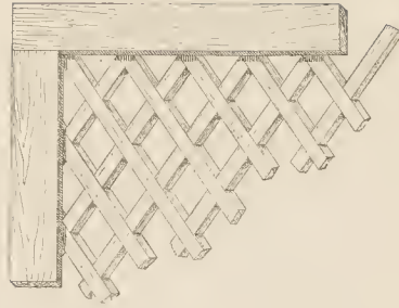
Fig. 72. Holzverbindung.
