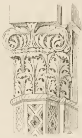
Fig. 102. Capitael aus der Moschee in Cordova X. Jahrs.
