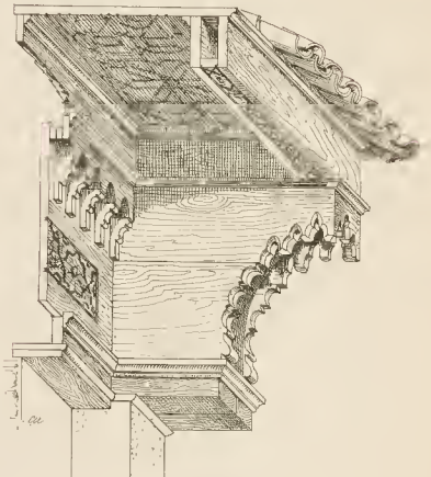
Fig. 95. Vom Portal der Moschee in Tanger (Afrika).
