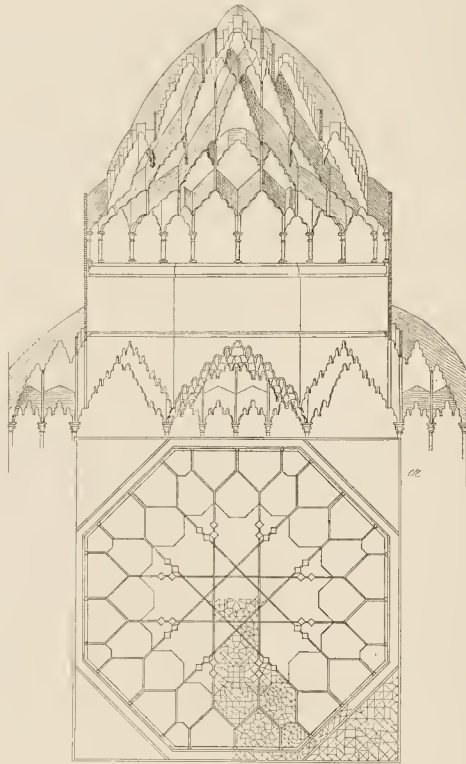
Fig. 88. Grundriss und Diagonalschnitt zum Bohlengerüst des Stalactitengewölbes im Saal der beiden Schwestern in der Alhambra.
