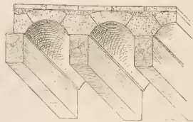
Fig. 64. Decke in Valencia.
