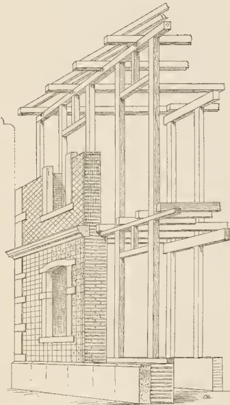
Fig. 52. Moderner Fachwerksbau in Lissabon.
