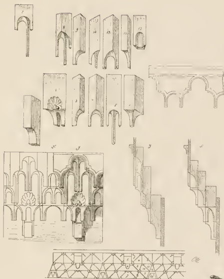
Fig. 89. Stucktongesims aus Holzbohlen im Museum der Alhambra.
