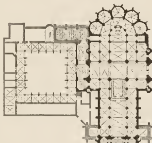
Fig. 117. Kathedrale von Leon, erb. 1250—1300.
