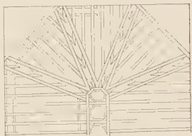
Fig. 68. Decke im Obergeschoss des Hotel Madrid in Sevilla.
