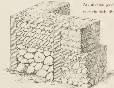
Fig. 37. Mauerwerk der Alhambra.
