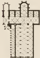
Fig. 115. Cluniacenser Klosterkirche Las Huelgas bei Burgos, erb. 1180—1182.
