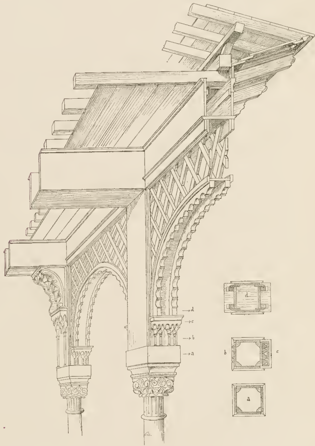
Fig. 99. Urspruengliche Holzconstruction des Loewenhofes in der Alhambra.
