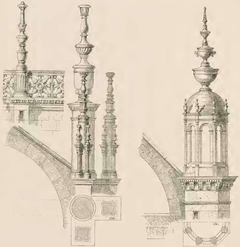
Fig. 133. Renaissanceaufbauten auf gothischen Strebeepfeilern der Cathedrale von Leon 1530—1550.
