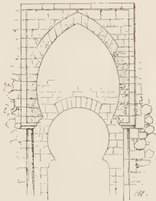
Fig. 43. Bogen der Puerta del Sol in Toledo.
