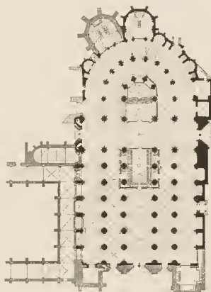
Fig. 117. Kathedrale von Toledo, begonnen 1227, Westfront 1426—1479, Kreuzgang Ende XIV. Jahrh.
