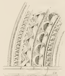
Fig. 125. Thuerbogen der Cathedralen von Valencia.
