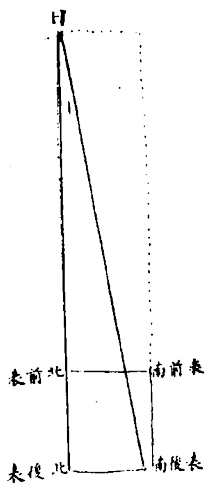
圖例比股勾遠日測
