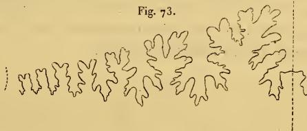
Desmoceras pyrenaicum (gros. = 10), d'après l'échantillon représenté pl. XXXVII, fig. 9. (Clichés de M. Nicklès.)
