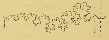
Platiceras syrtale (gros. = 3,5), d'après l'échantillon représenté pl. V, fig. 3.
