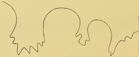
Tissotia Ewaldi (gros. = 3,3), d'après l'échantillon de la craie de Villedieu, représenté pl. IV, fig. 6.
