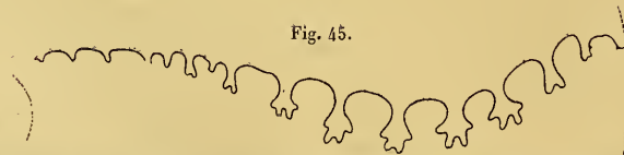
Sphenodiscus cf. pedernalis (gros. = 2,5), dessin de M. Douvillé, d'après un échantillon de Sainte-Croix, près le Mans.
