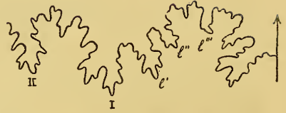
Sonneratia Cleon (gros. = 4,5), d'après Douvillé, B. S. G. F., 3 e , XVIII, p. 289.
