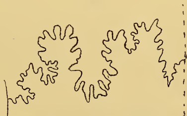
Gauthiericeras bajuvaricum (gros. = 4,30), d'après l'échantillon représenté pl. XII, fig. 3.
