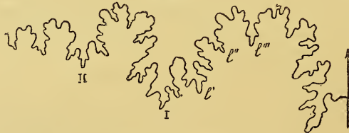
Hoplites splendens (gros. = 4,5), d'après Douvillé, B. S. G. F., 3 e , XVIII, p. 289.
