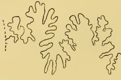
Peroniceras Moureti (grand. nat.), d'après un échantillon de la craie de Villedieu.
