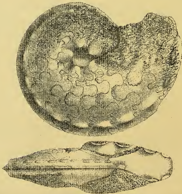
Tissotia Slizewiczi , reproduction de la figure donnée par M. Fallot, Crétacé . . . . pl. II, fig. 2.
