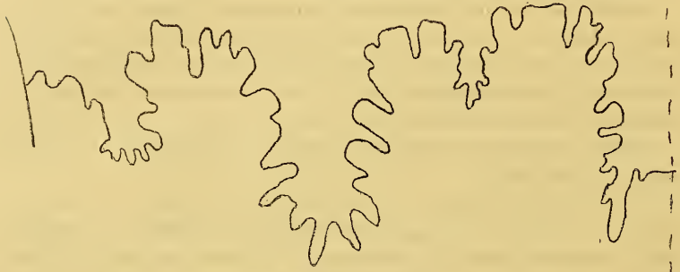
Mortoniceras Bontanti (gros. = 3), d'après l'échantillon de la craie de Villedieu représenté pl. XVII, fig. 3.
