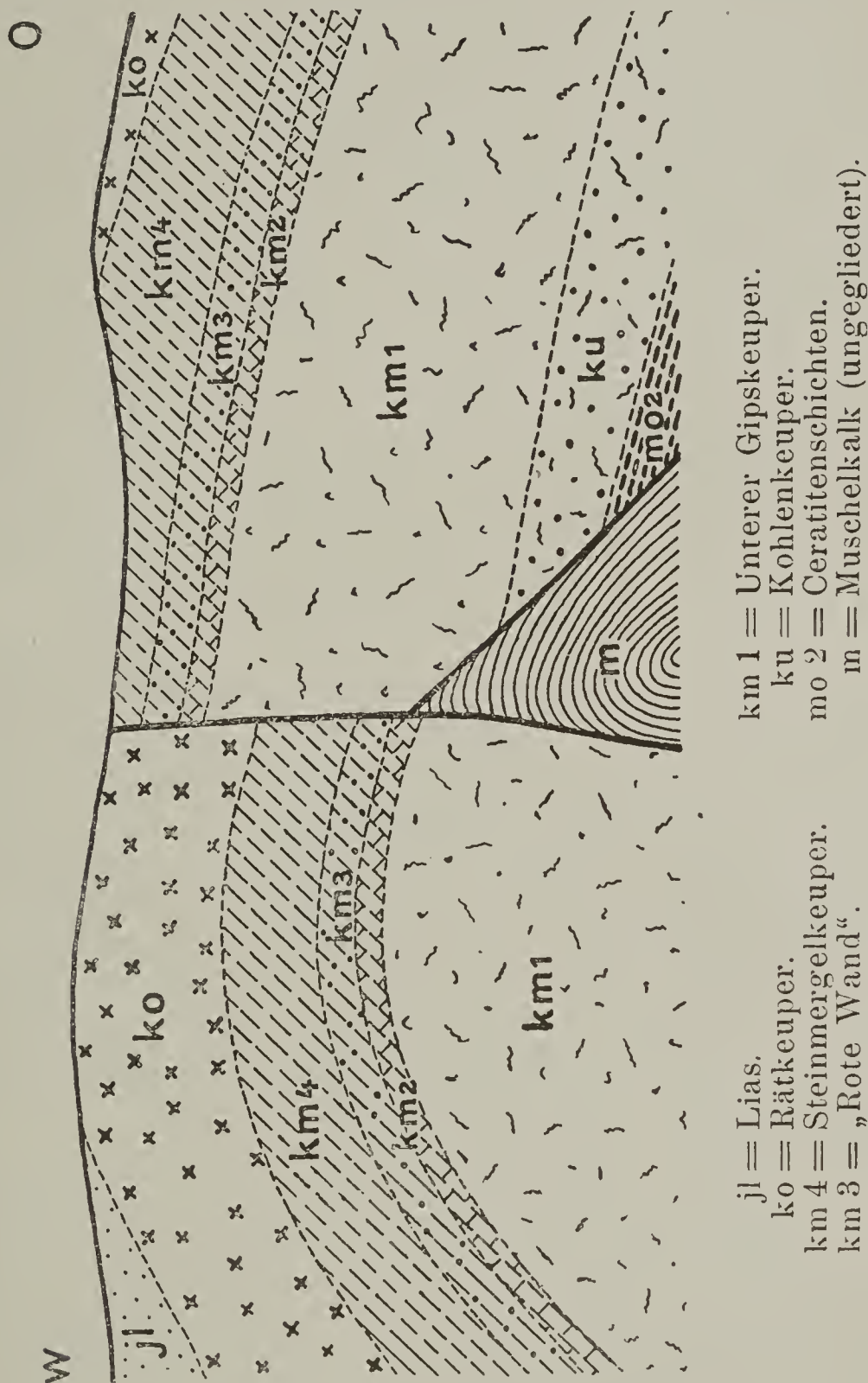
Fig. 3. Verallgemeinertes Profil durch die Schichten zu beiden Seiten der Oeynhaus. Vlothoer Hauptstörung.
