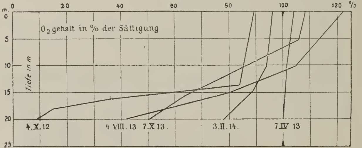
Kurventafel II. Schalkenmehrener Maar. Sauerstoffschiehtung.
