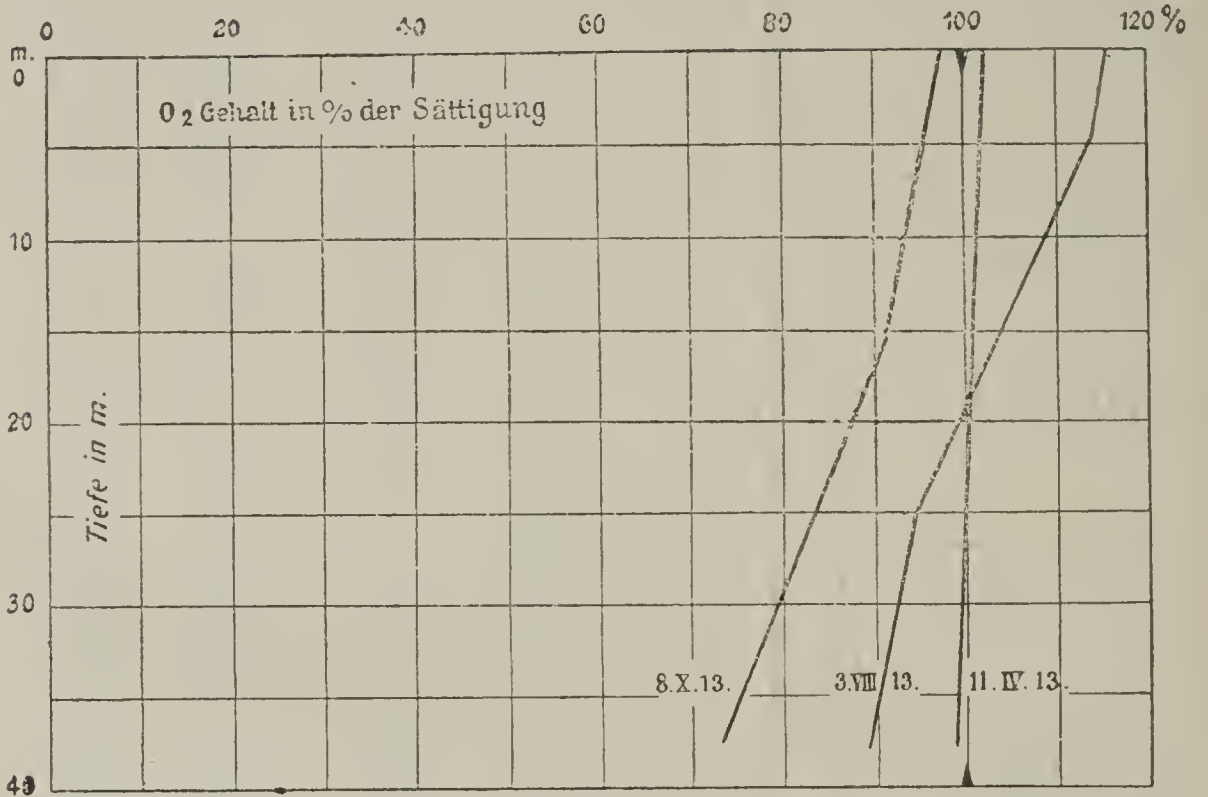
Kurventafel I. Gemündener Maar. Sauerstoffschiehtung.
