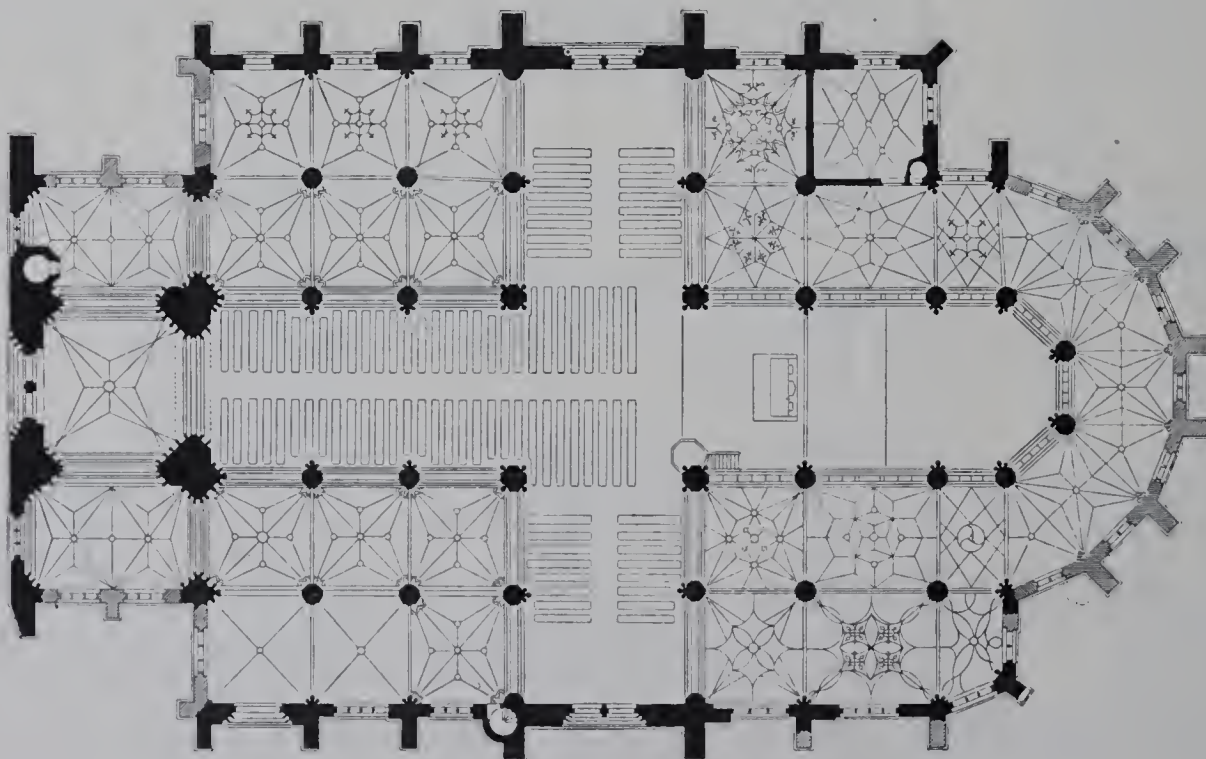
Oberer Grundriss.
