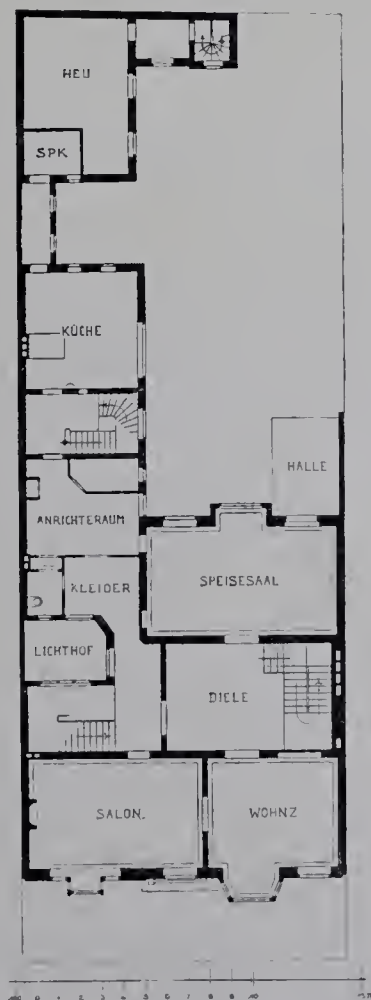
Hauptgeschoss.
