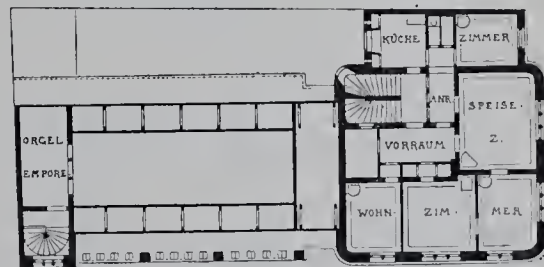
IV. Stockwerk.
