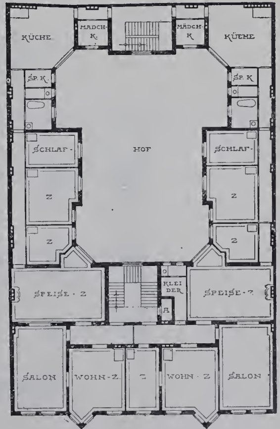
II. Stockwerk.
