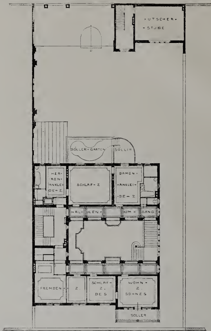
Obergeschoss.
