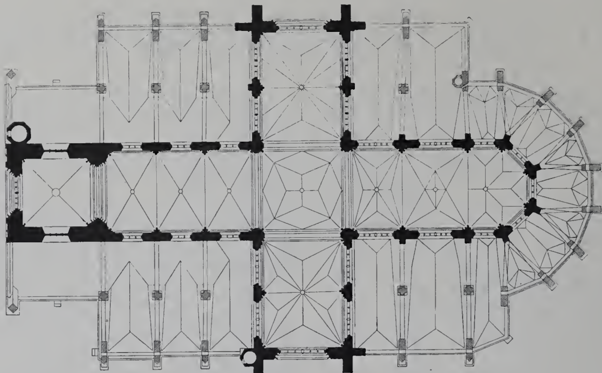
Oberer Grundriss.
