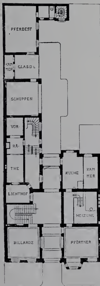
Untergeschoss.
