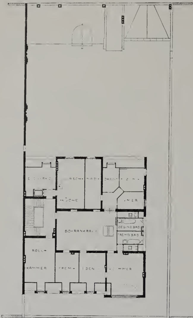
Dachgeschoss.
