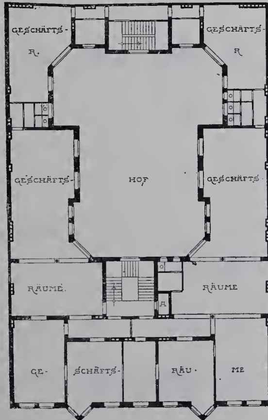
I. Stockwerk.
