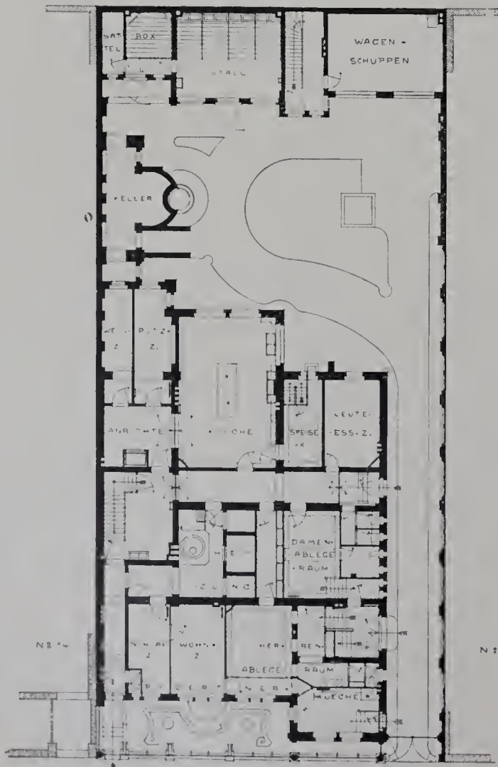
Untergeschoss.
