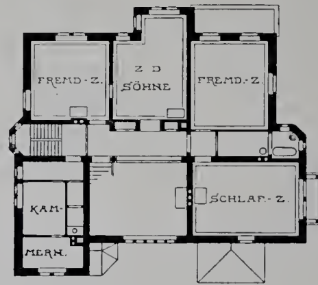
Obergeschoss.
