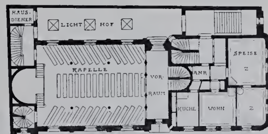
II. Stockwerk.
