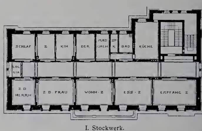
I. Stockwerk.
