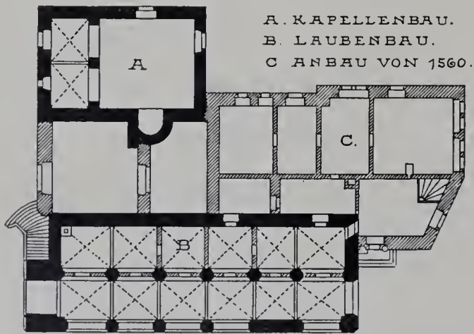
Untergeschoss.
