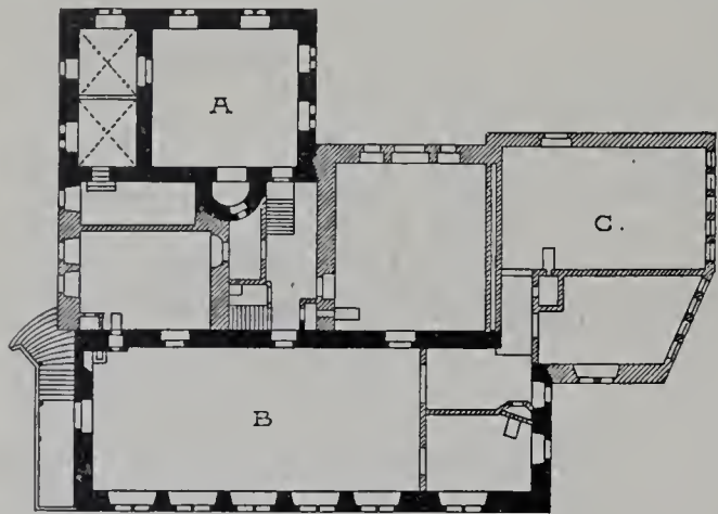
Obergeschoss.
