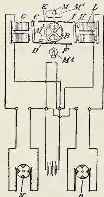
THE RENFAX SYNCHRONIZER
