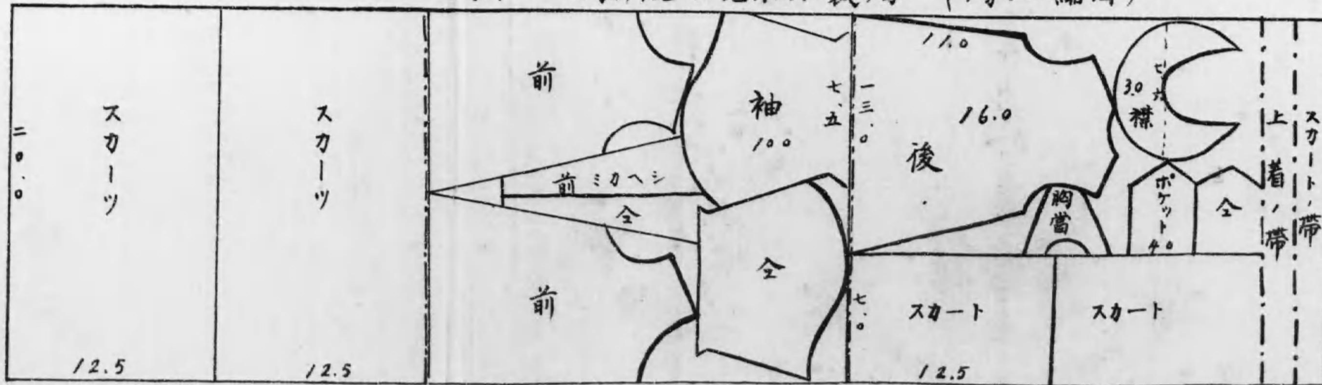
二尺幅ノ中裁袴ニテ十歳前後ノ女児水兵ノ裁方(十分ノ一縮図)
