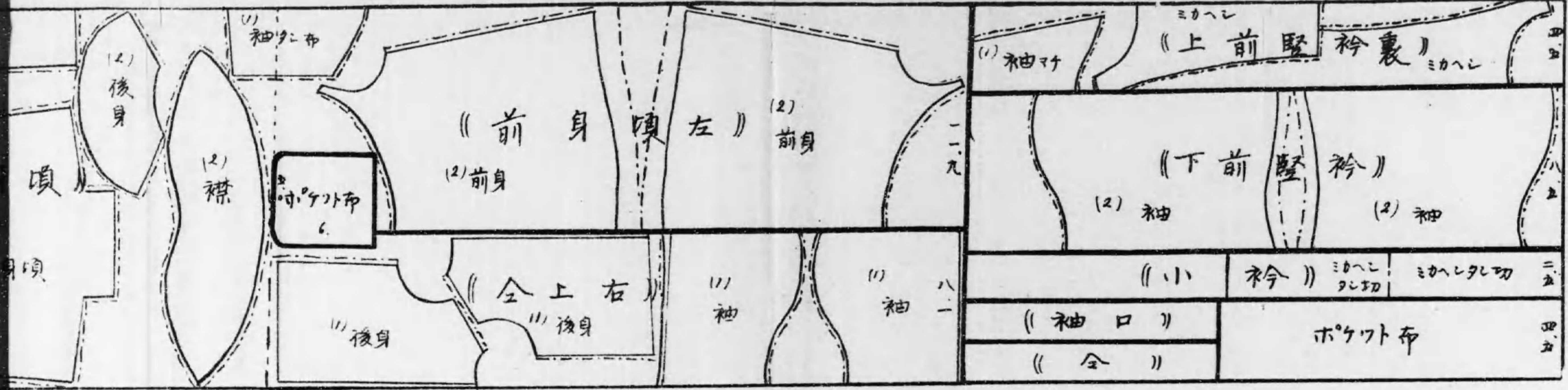
コートを利用して八九歳の女児服及び外套の裁合せ図 (十分の一縮図)
