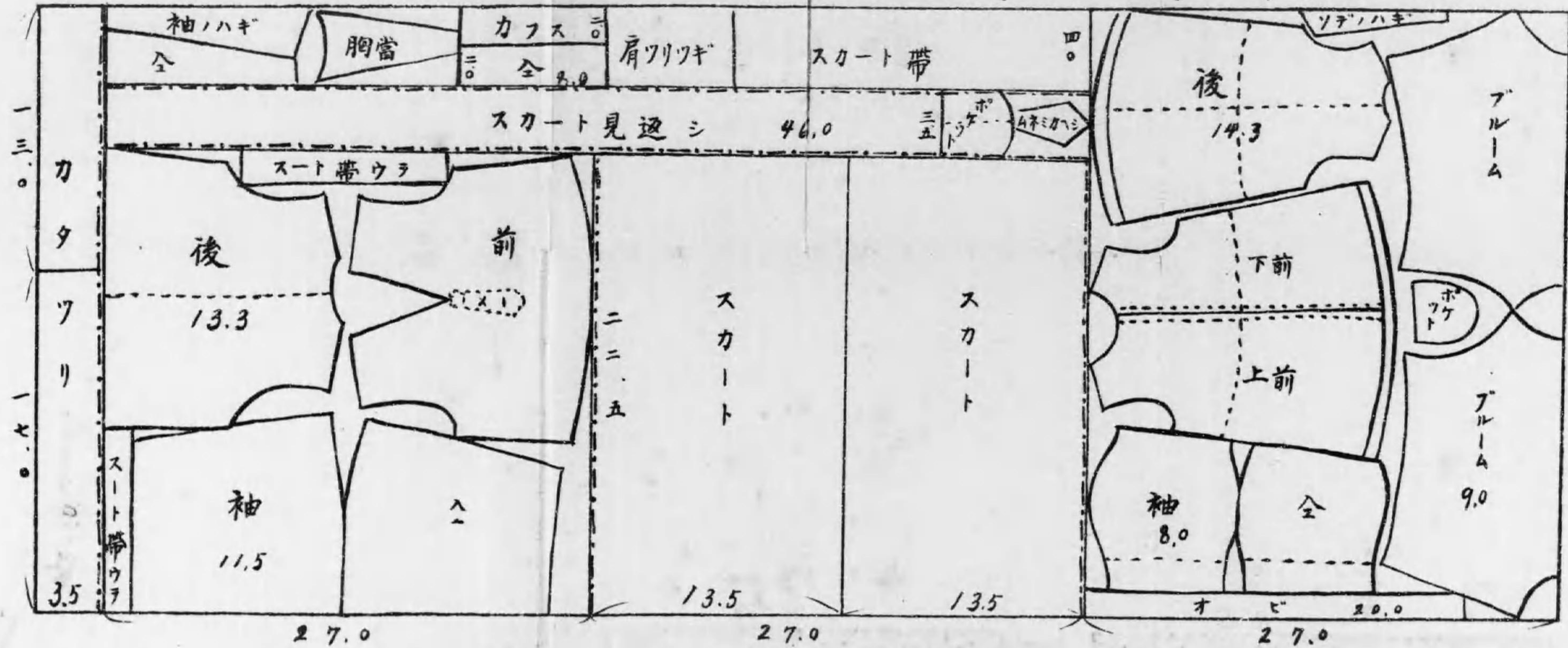
三尺幅女袴ニテ十二歳女児帯ナシセラー(襟ハ別布)及び五歳女児スート裁合せ圖(十分ノ一縮図)
