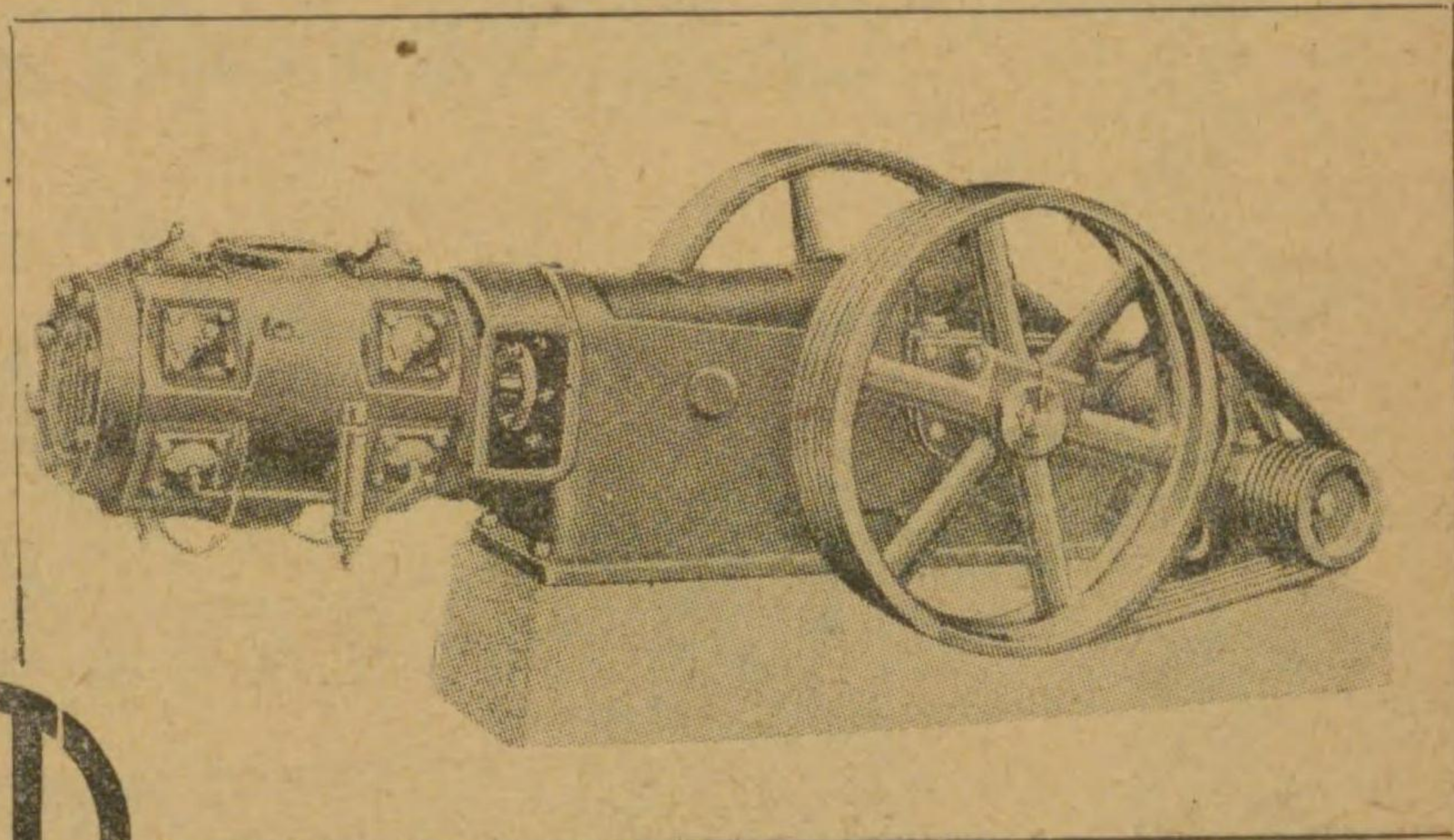
二段壓縮空冷式
