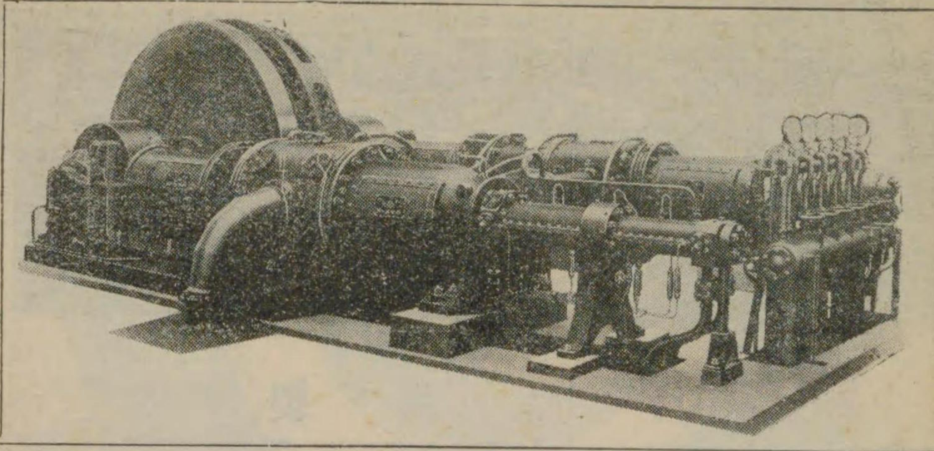
神鋼横型六段瓦斯壓搾機
