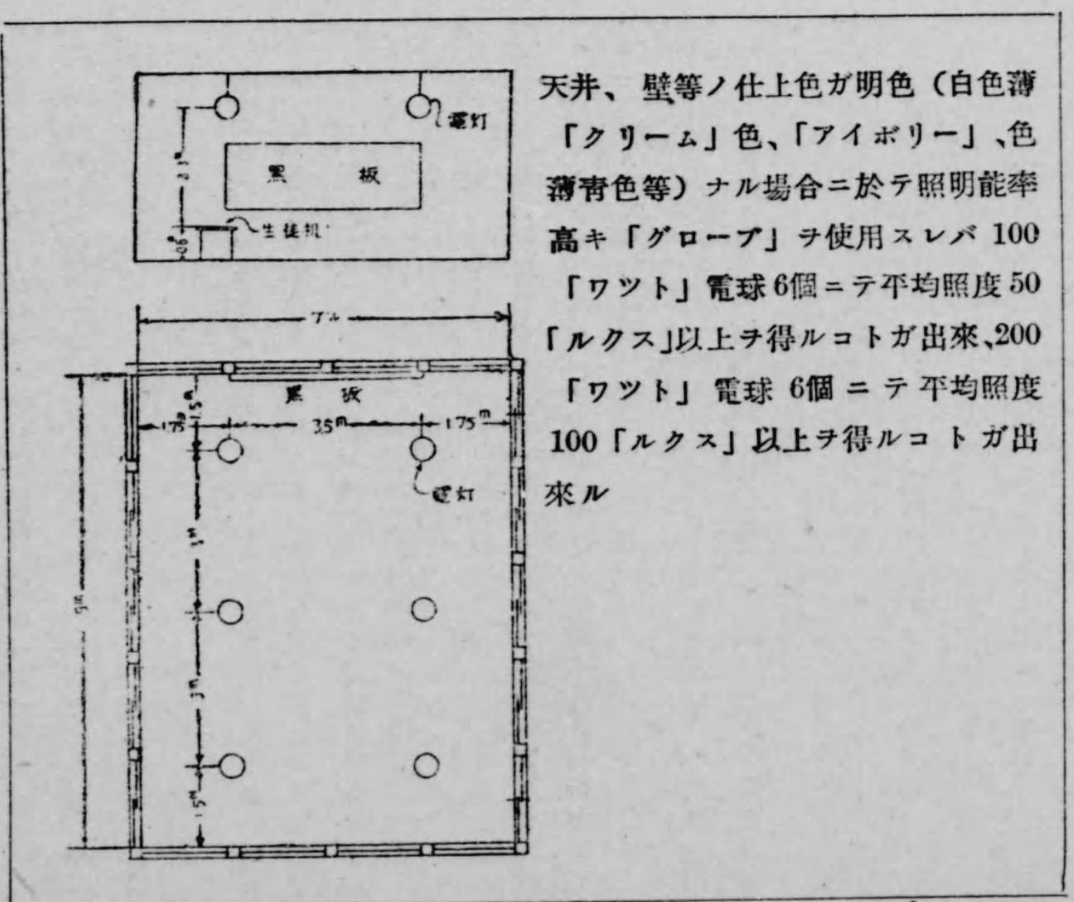
教室照明施設例
