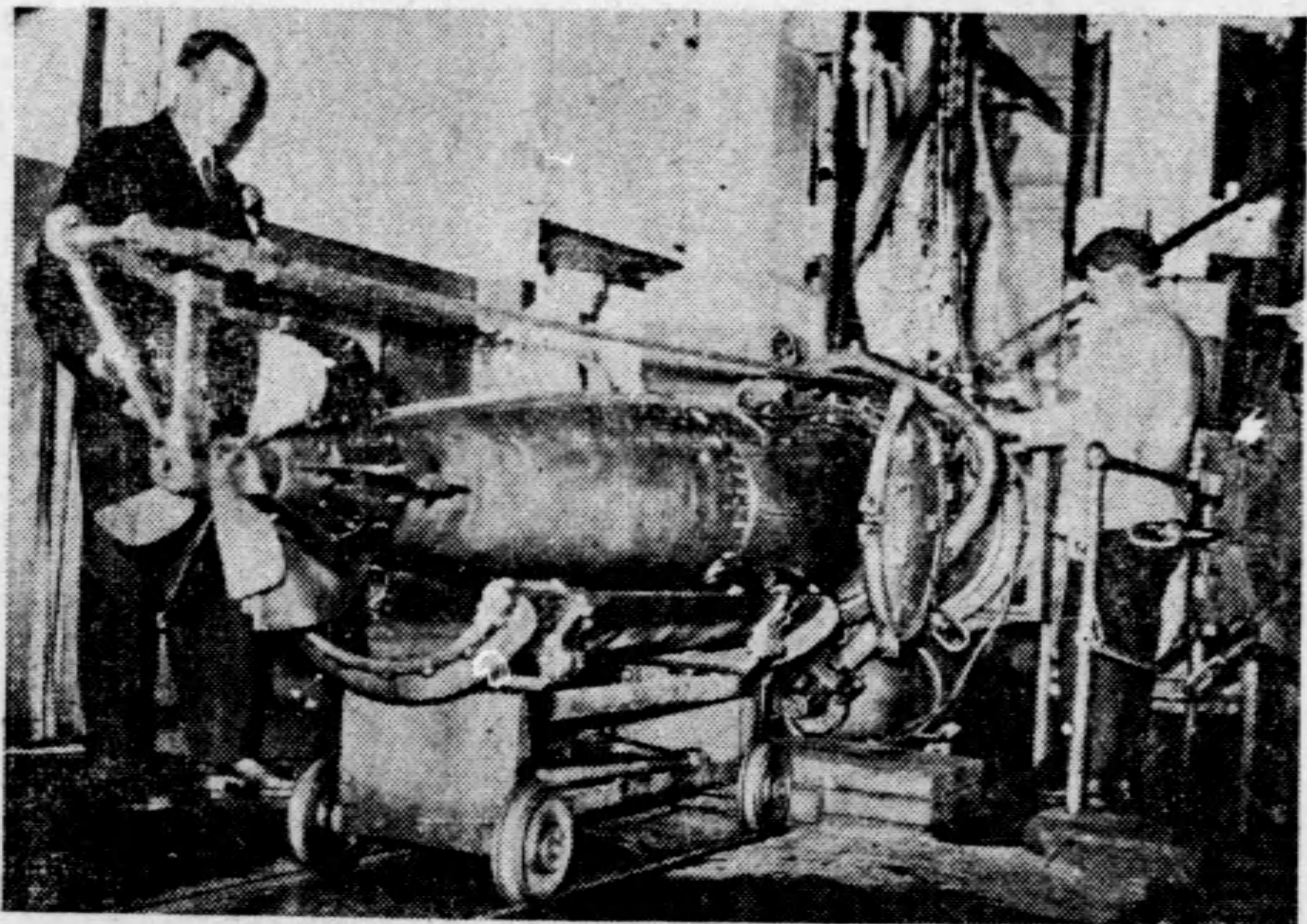
魚雷之全貌 此種魚雷，可沉三萬五千噸，戰艦之圖示，製造完成，裝入試驗管，審查情形。
