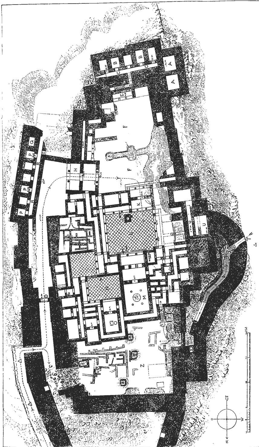
Планъ «верхняго города» въ Тирисѣ, составленный Дѣрифельдомъ: —А. Башня съ двумя комнатами. —В. Помѣщеніе со сводами —С. Галерея. — Д. Корридоръ съ лестницей. —Е. Колоннада. —F. Главный передній дворъ. —G. Юго-западный уголъ двора. —H. Большіе Проилеи. —I. Коло- нада. —K. Малые Проилеи. —L. Большой дворъ. —M. Помѣщеніе для мужчинъ. —N. Малый дворъ. —O. Помѣщеніе для женщинъ. —P. Помѣ- щеніе со сводами. —Q. Цистерна. —R. Галерея восточныхъ стѣнъ. —S. Шахта, выкопанная въ 1876 г. —T. Боковой подъемъ. —U. Мѣсто для подвала. —V. Цистерна. —W. Башня на сѣверо-западѣ. —X. Малая лестница. —Y. Входъ въ «средній городъ». —Z. Средній или задній дворъ. — 1. Башня на сѣверо-востокѣ. —А. Направленіе главнаго подъема. —В. Городскія ворота. —Л. Жертвенникъ на дворѣ. —Е. Мѣсто, гдѣ найдены терракотты. —Z. Дверь въ галерею K. —Ф. Стѣны.
