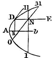
Parabola.
