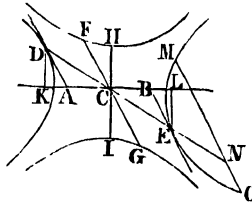
Hyperbolas.
