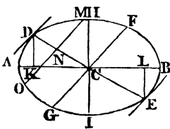
Ellipse.
