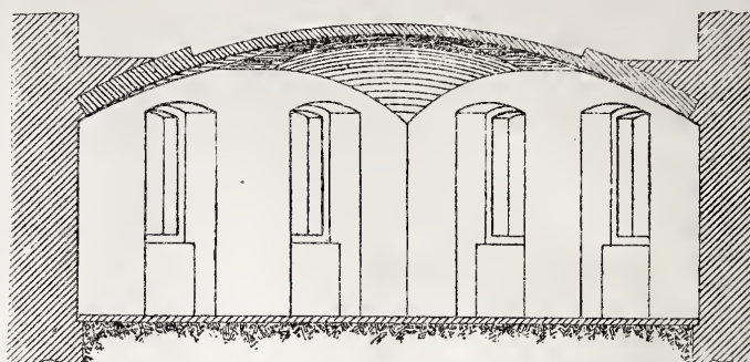
Schnitt c-d.
