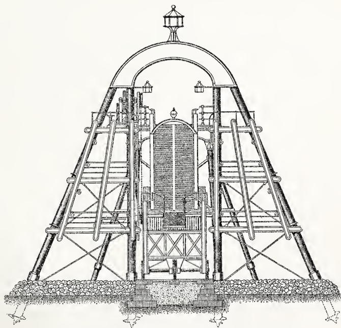
Landepier der Dampf-Fähre von Egremont bei Birkenhead.
