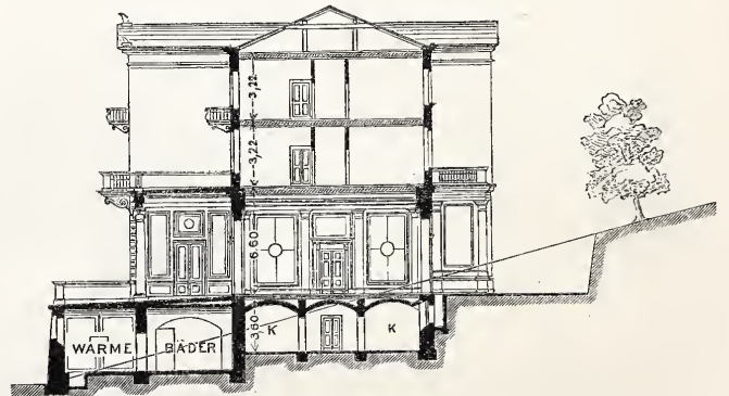
Durchschnitt.
