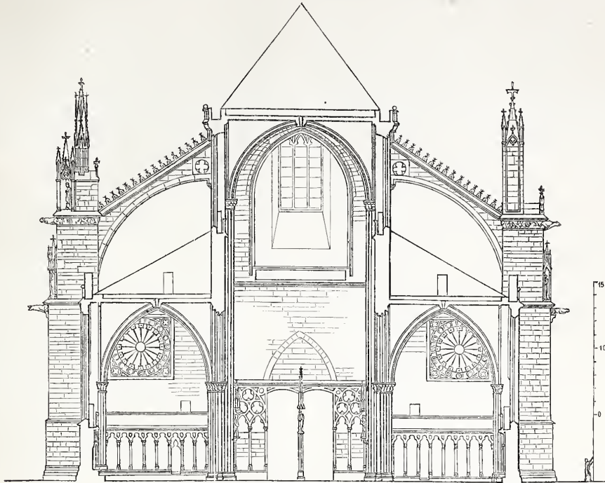
Fig. 4. Querschnitt mit der Ansicht nach Westen.
