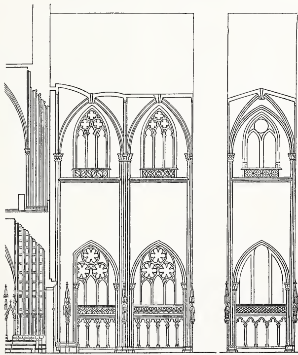
Fig. 6 u. 7. Systeme des Inneren. Westjoche. Ostjoche.
