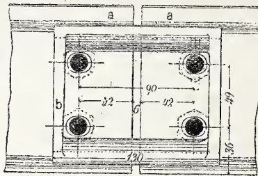
Fig. 6. Gussklotz am Schienenstofs.
