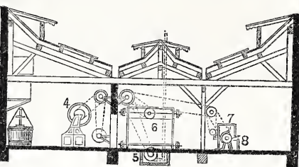
Durchschnitt durch das Waschhaus.
