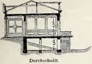
Durchschnitt.
