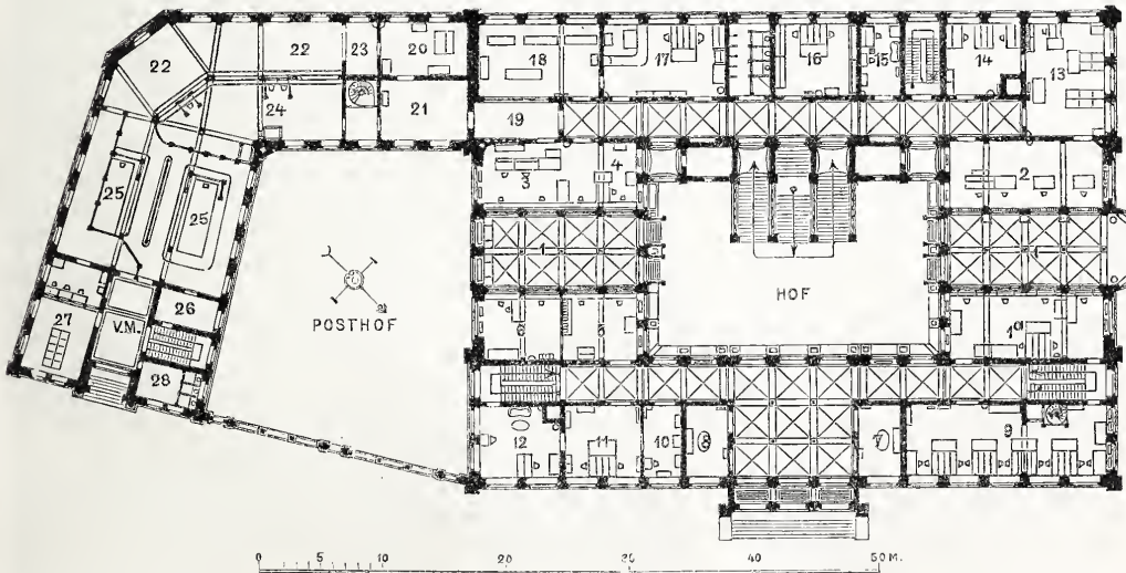
Post- und Telegraphen-Gebäude zu Bremen.
