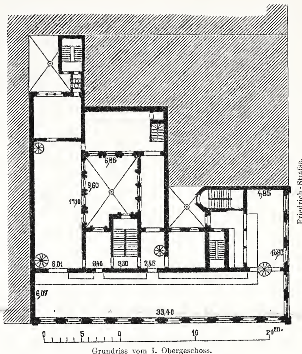
Grundriss vom I. Obergeschoss. Geschäftshaus von R. D. Warburg & Comp. in Berlin. Architekten von der Hude & Hennicke.
