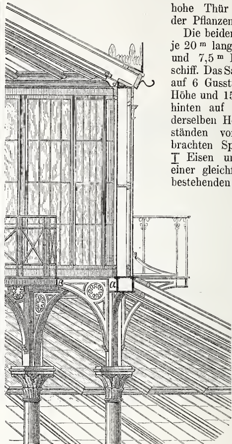
Details der Konstruktion des Palmenhauses.
