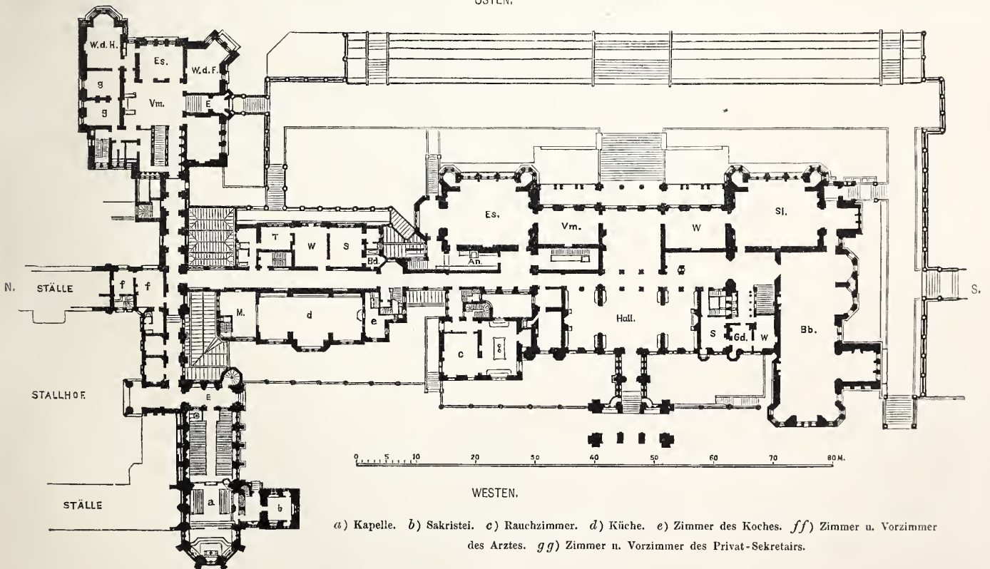
Grundriß vom Erdgeschoss.
