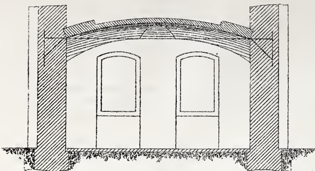
Schnitt a-b.
