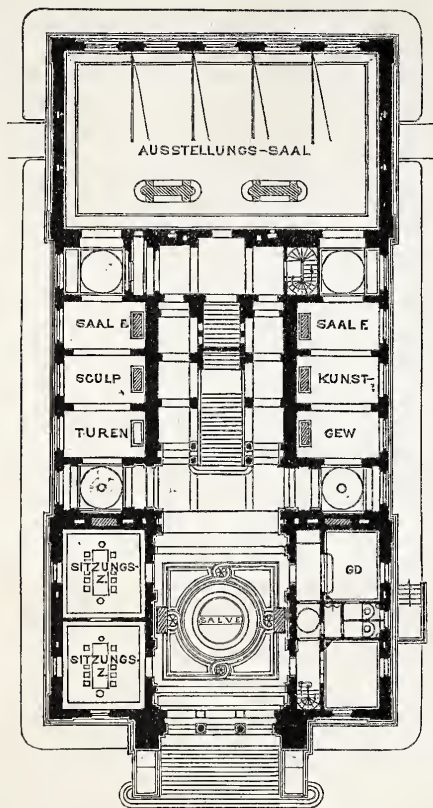
Untergeschoss.
