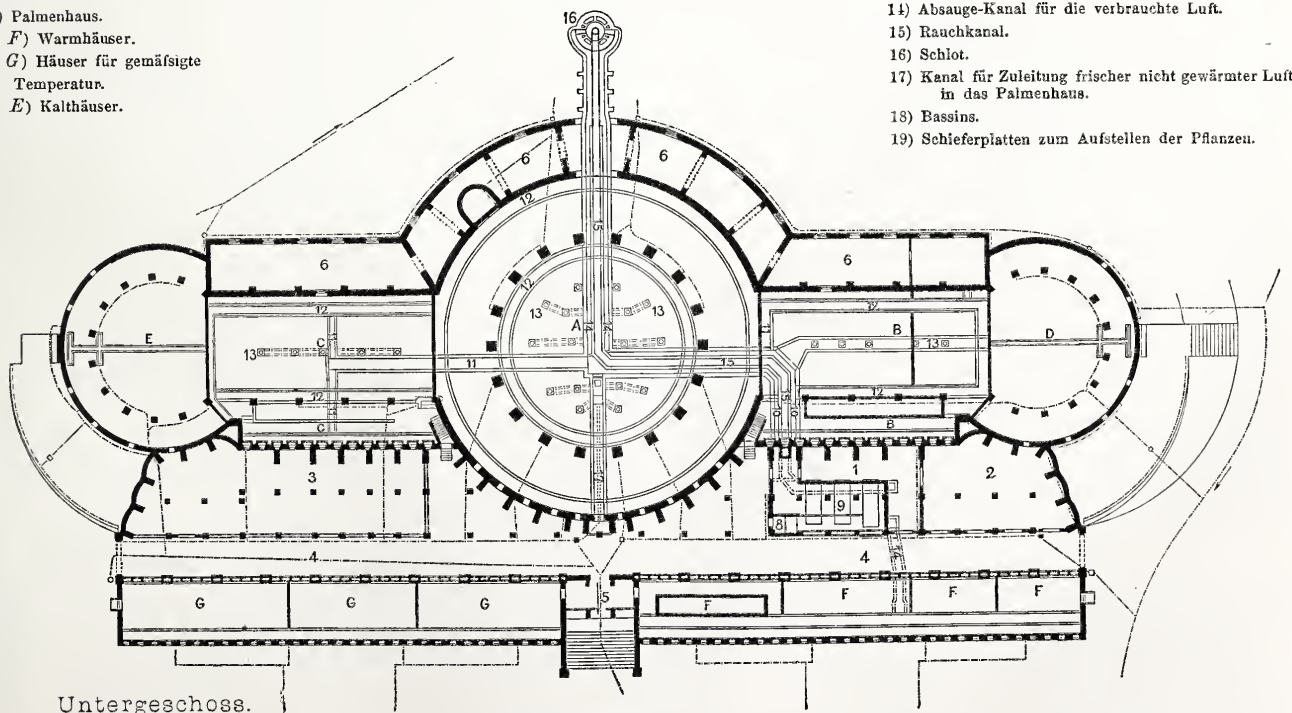
Untergeschoss.
