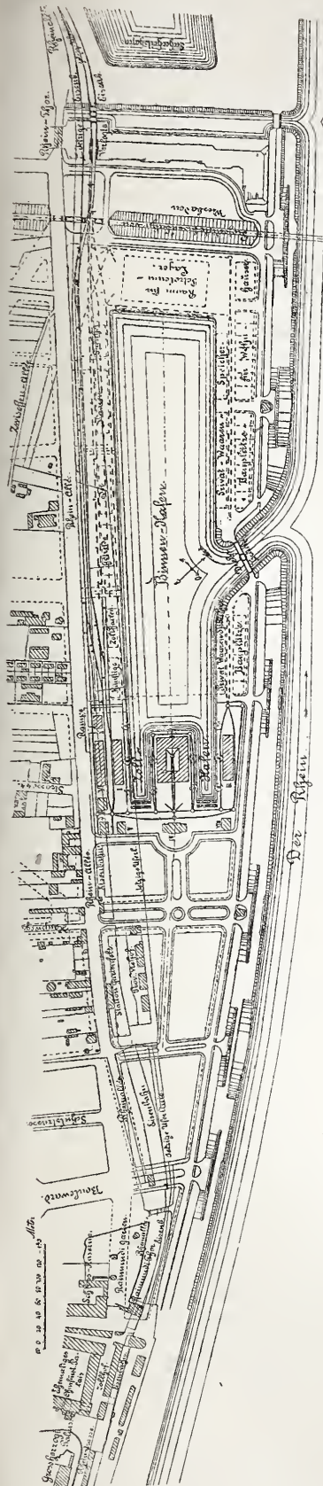
PROJEKT ZUR ANLAGE EINES ZOLL- UND BINNENHAFENS BEI MAINZ.
