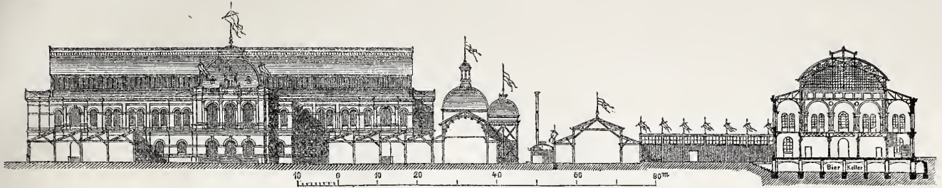
Längenschnitt
