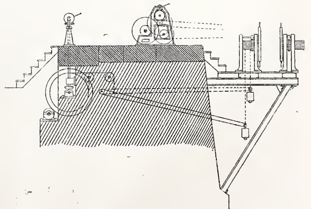
Patentirter Kohlenkipper von Gerhardt.
