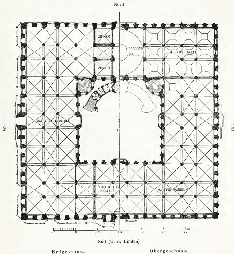
Umbau des Zeughauses zu Berlin. (Arch. F. Hitzig)
