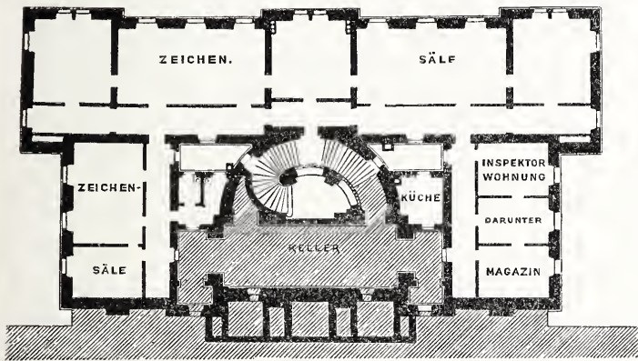
Untergeschoss.
