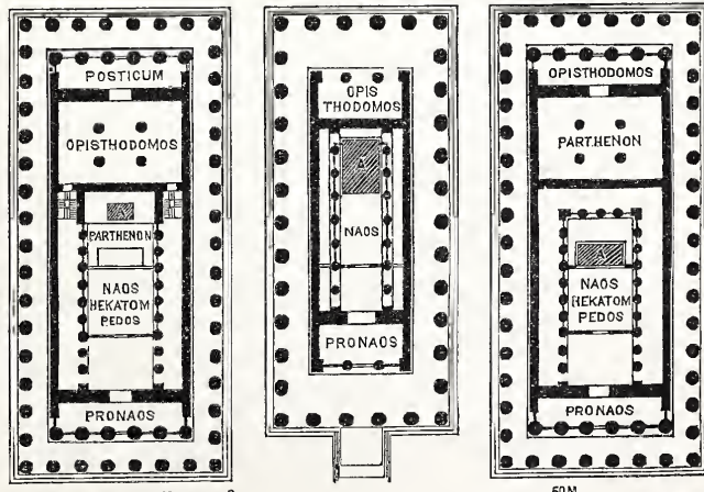
Parthenon nach C. Bötticher. Zeustempel in Olympia. Parthenon nach Penrose.
