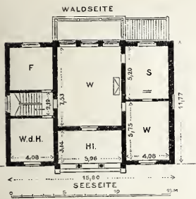
Grundriss.
