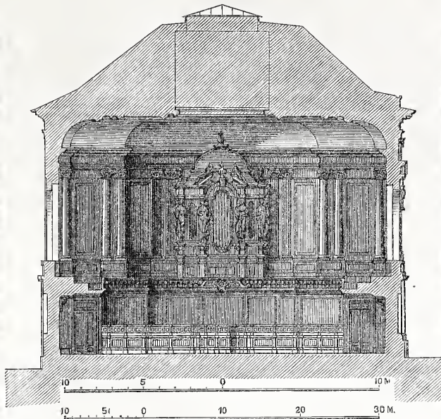
Musiksaal in Basel.
