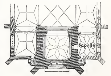
Grundriss des Neubaues.
