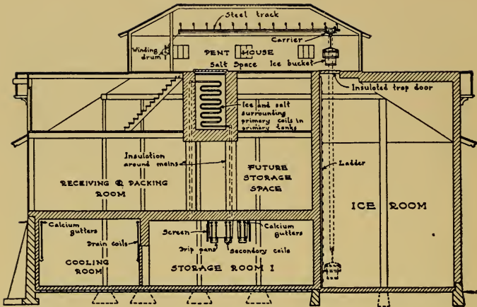
LONGITUDINAL SECTION
