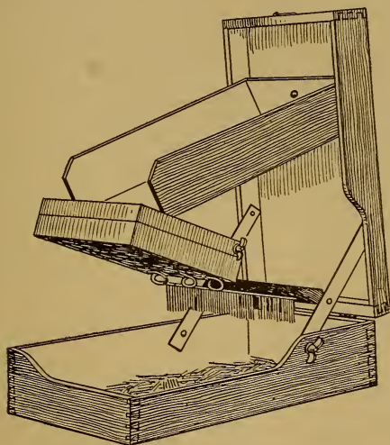
Fig. 72.—“NAIL STRIPPER”
