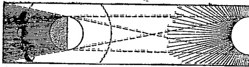
月 蝕
