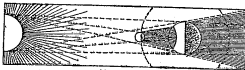
日 蝕
