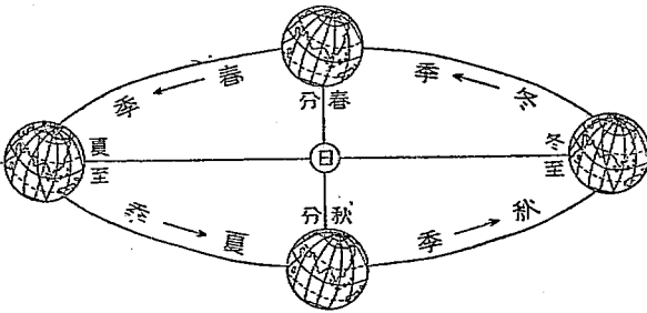
地球公轉和四季
