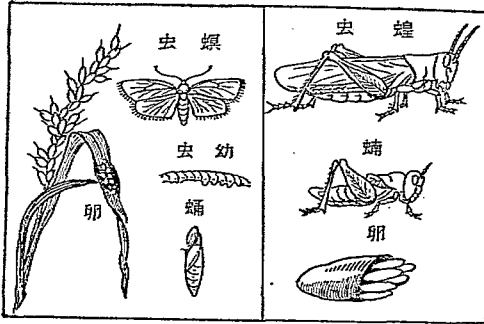
長生的蟲螟
