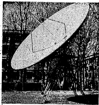
中国科学院科学仪器厂在有关单位协作下，自行设计并研制成功一台LT-1型扫描干涉仪，填补了我国干涉仪的空白，为我国赶超世界科学技术先进水平作出了贡献。
