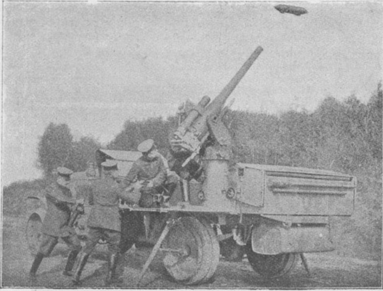
Германская пушка для стрѣльбы по воздухоплавательнымъ аппаратамъ.
