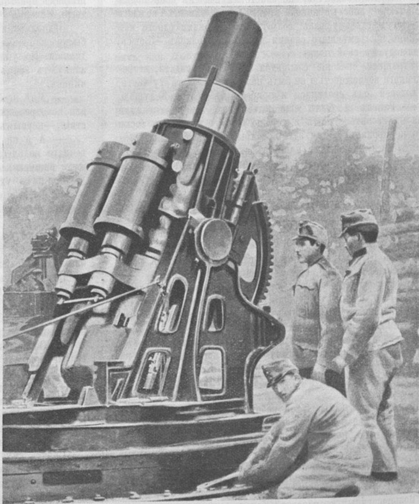
12-дм. австрійская гаубица. („Ill. London News“).
