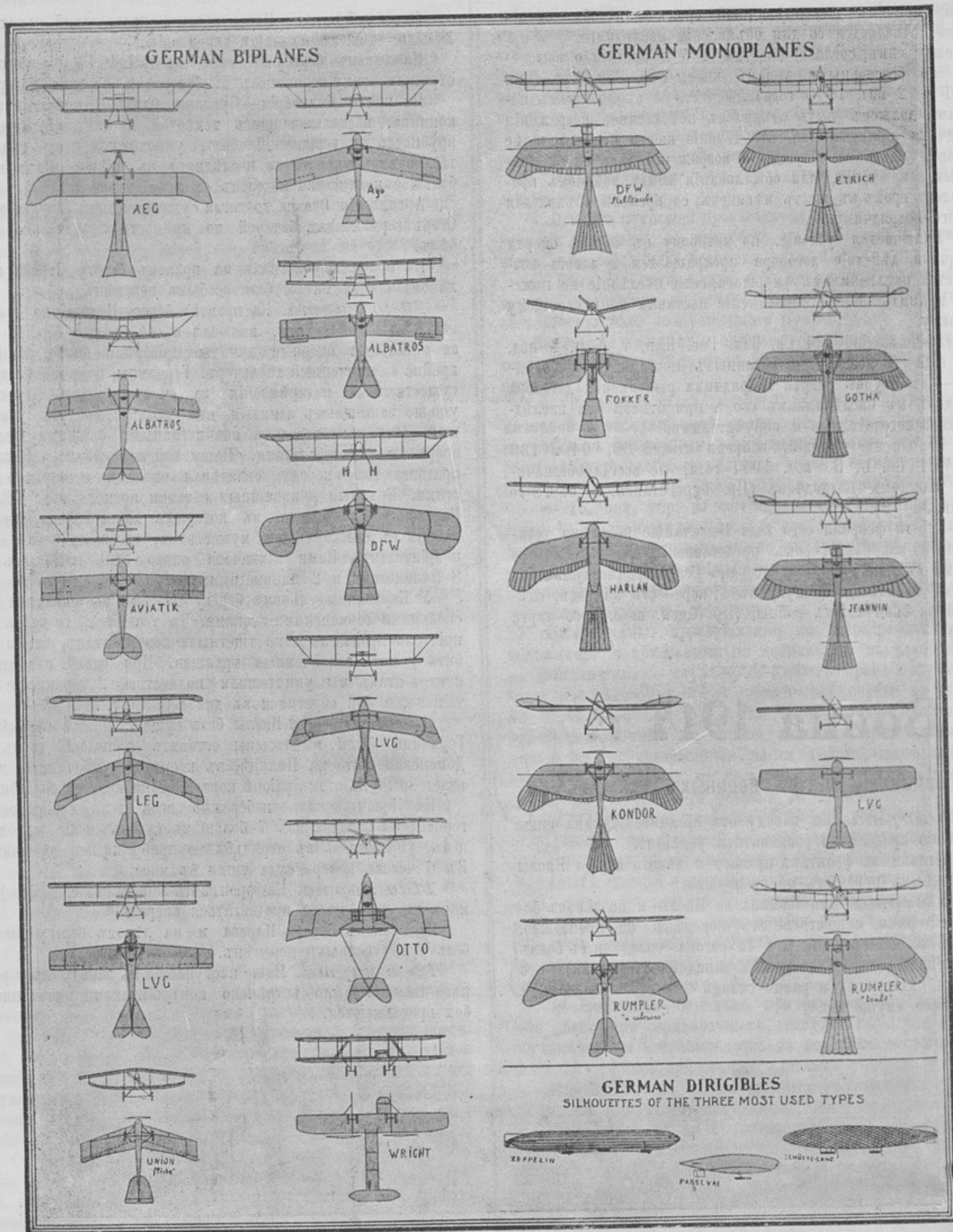
Типы германскихъ аэроплановъ. („Ill. London News“).
