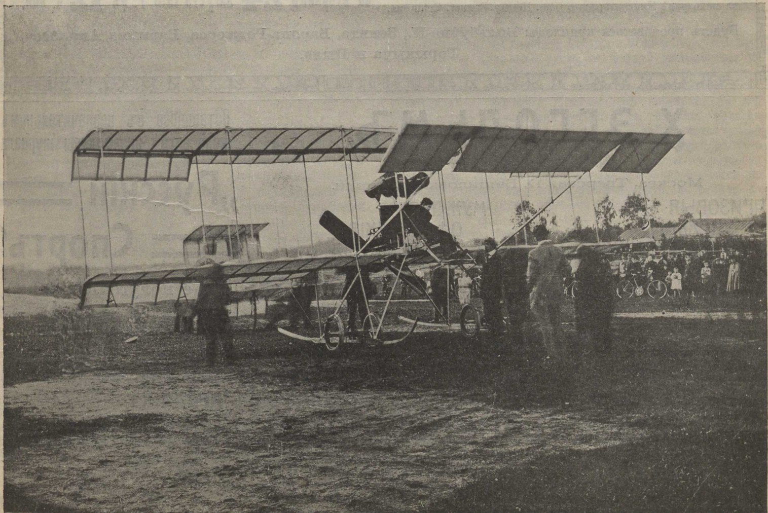
С. И. Уточкинъ на первомъ русскомъ бипланѣ, построенномъ на заводѣ „Дух“ Ю. А. Меллера въ Москвѣ.
