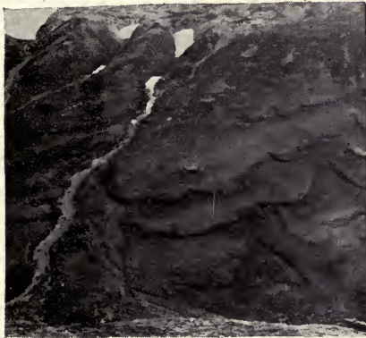
FIG. 162.—Sheet wash, Alaska. (Moffit, U. S. Geological Survey.)
