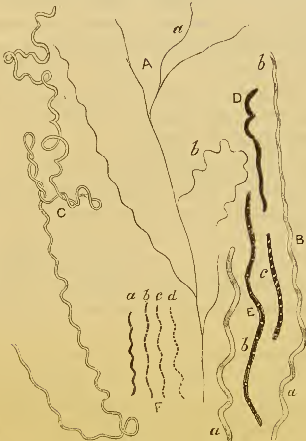
FIG. 129.—CLADOTRIX DICHOTOMA.
