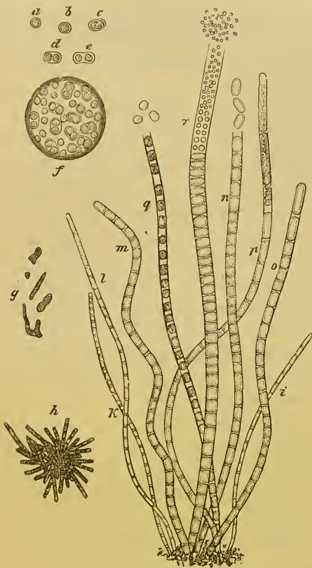
FIG. 126.—CRENOTHRIX KÜHNIANA.
