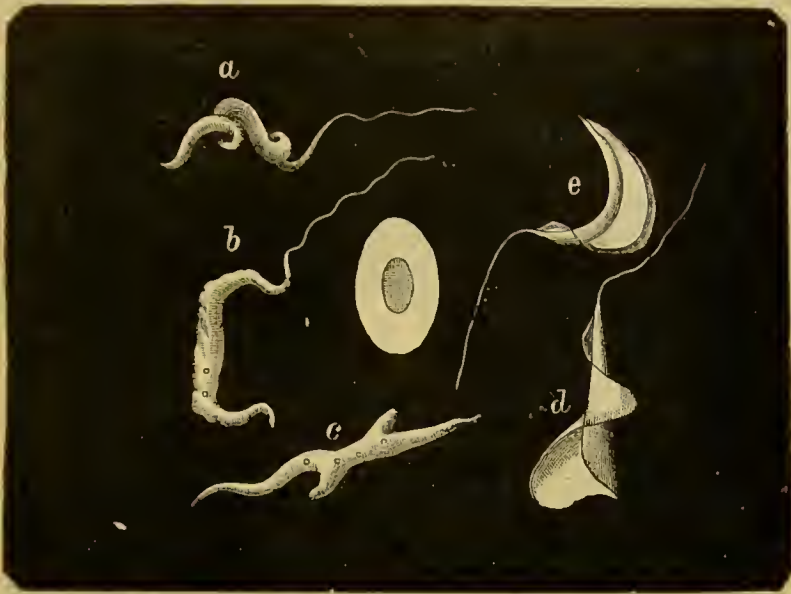
FIG. 131.—HEMATOMONAS COBITIS.
