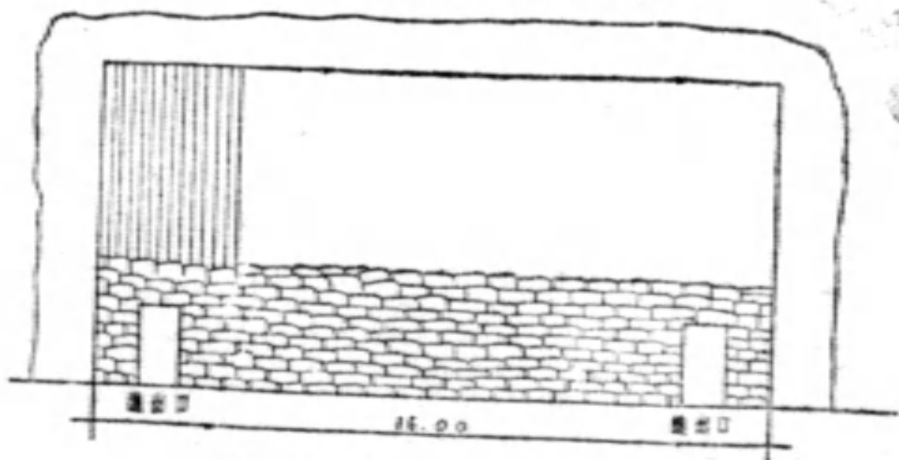
長形避難所正面圖 防禦百公斤炸彈可容七十人避難
