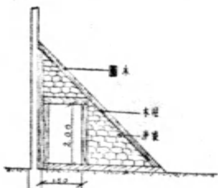
斷面圖
