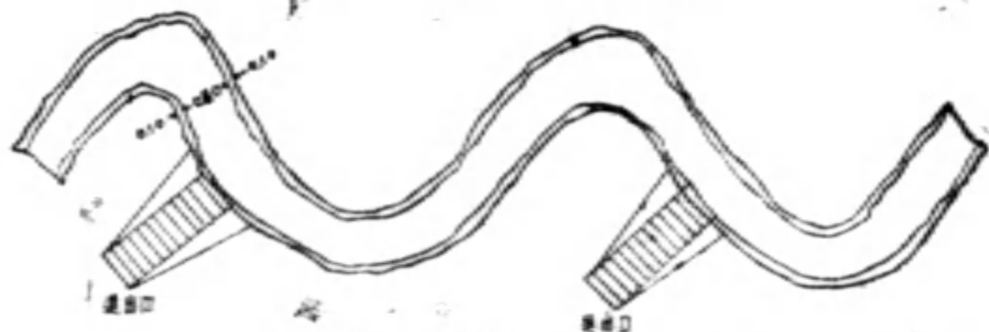
波浪防空壕平面圖 防禦破片每公尺可容二人
