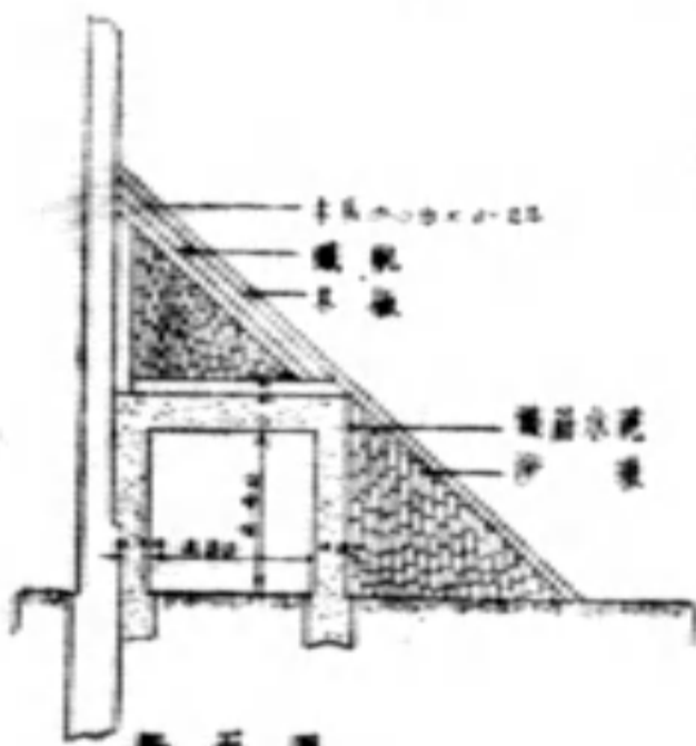
斷面圖
