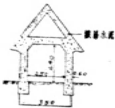
斷面圖
