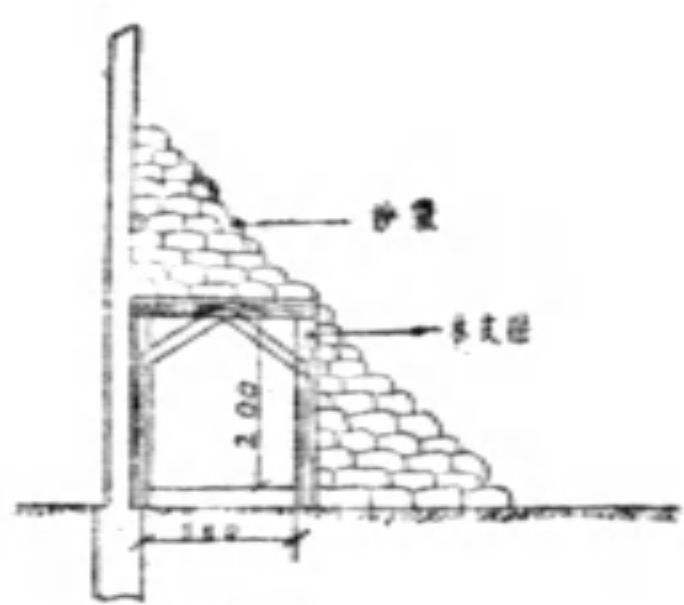
斷面圖
