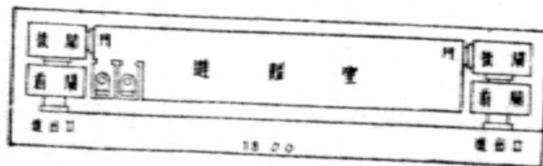
方形避難所平面圖 防護五十公斤炸彈可容六十人避難
