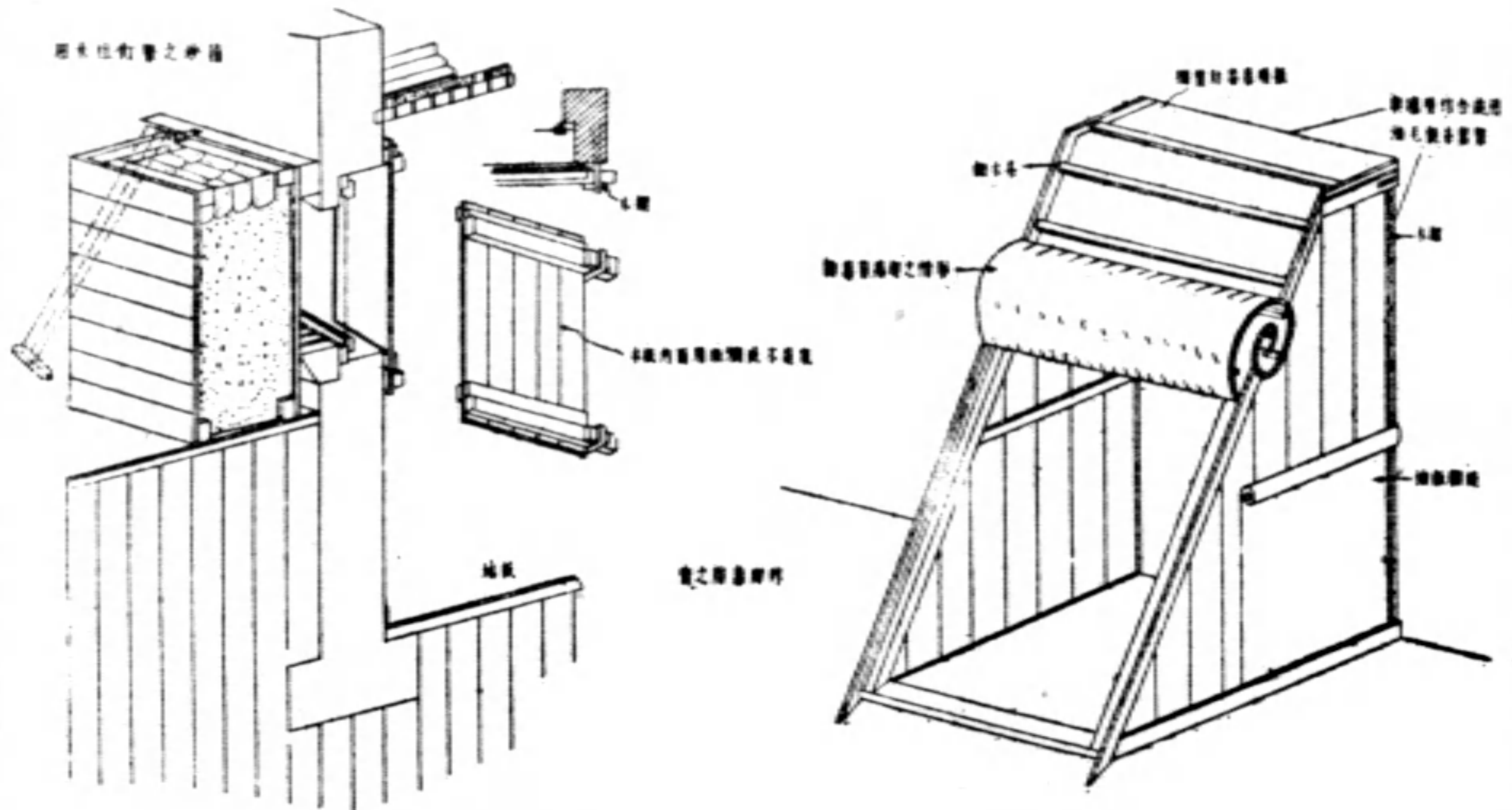
(丙) 窗戶防破片工事圖(一)
