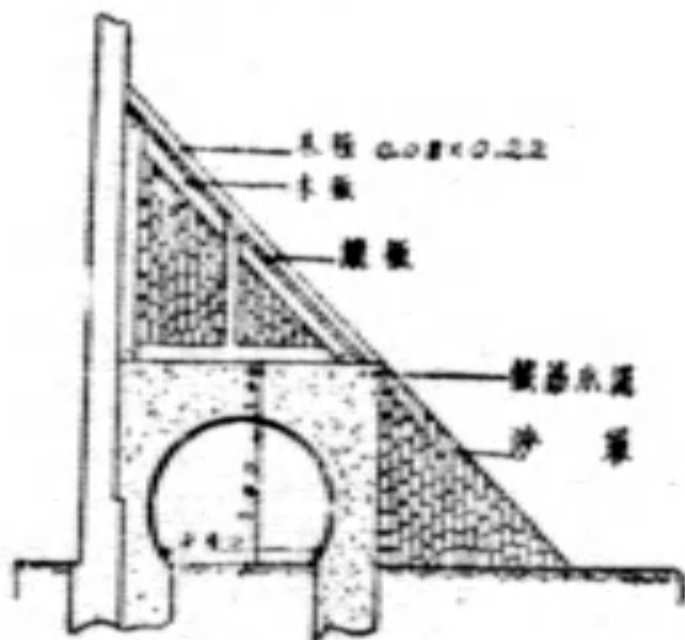
斷面圖
