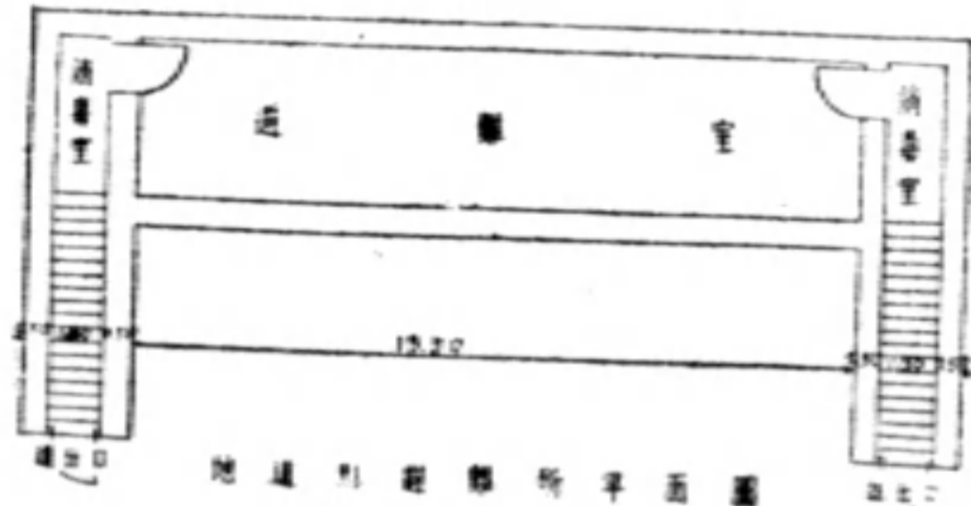
間隔之避難所平面圖 防護五十公斤炸彈可容一百二十人避難
