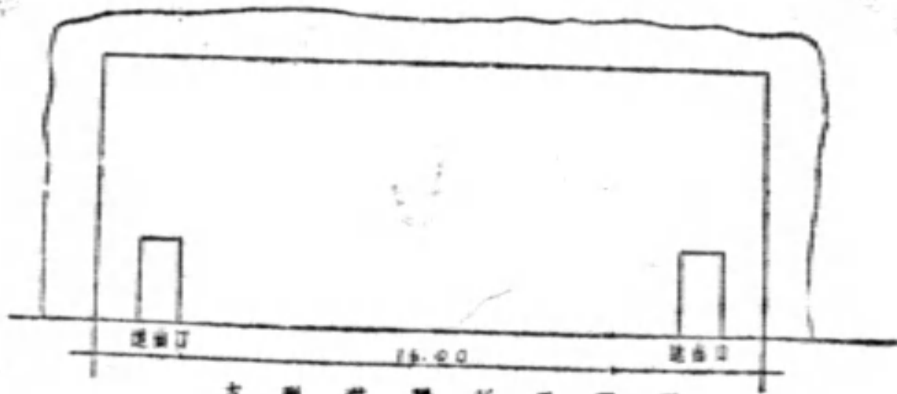
方形避難所正面圖 防禦五十公斤炸彈可容七十人避難
