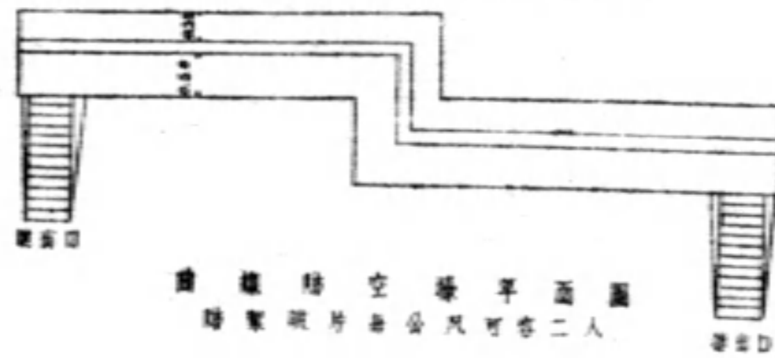
城壕防空壕平面圖 防禦破片每公尺可容二人
