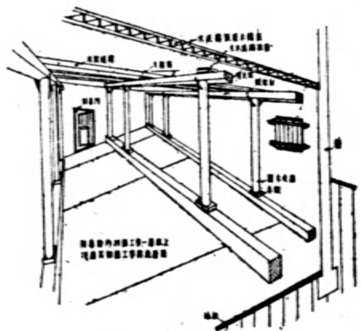
(乙) 普通房屋底層支撐作避難所圖形
