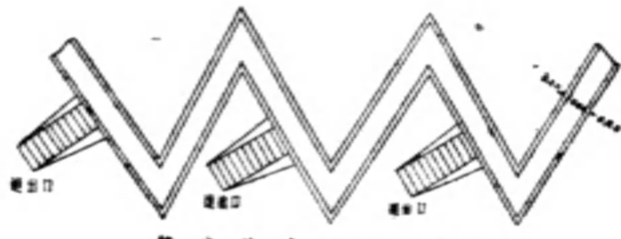
鋸齒防空壕平面圖 防禦破片每公尺可容二人
