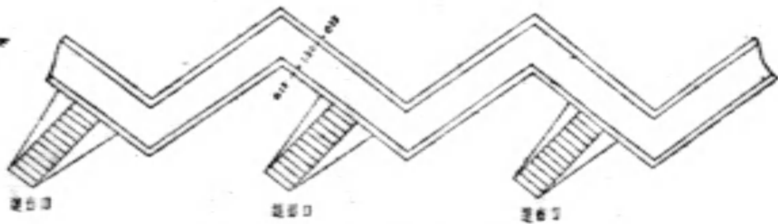
龜孔防空壕平面圖 防禦破片每公尺可容四人
