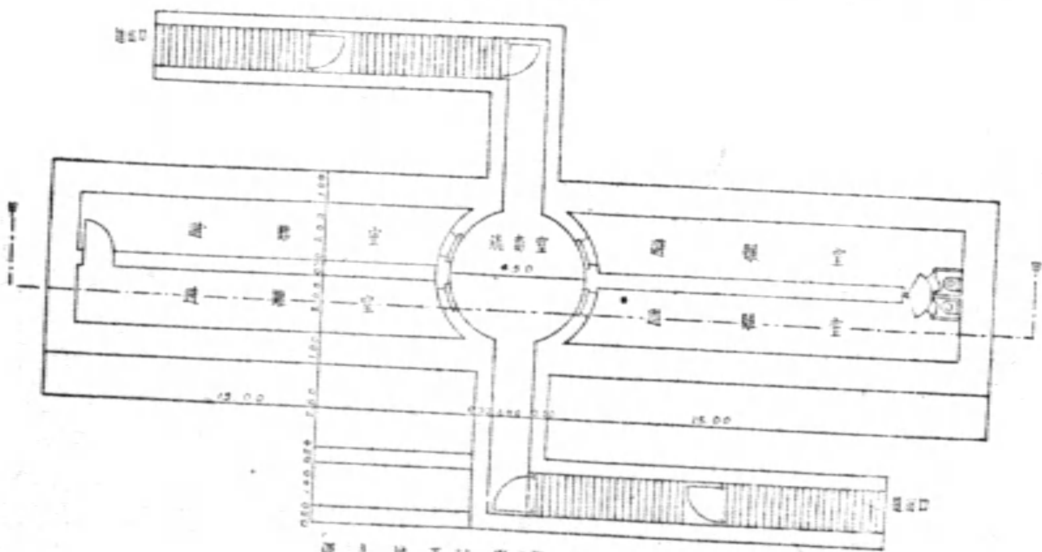
深入地下大型避難所平面圖 每室三百公斤炸彈可容二百人避難
