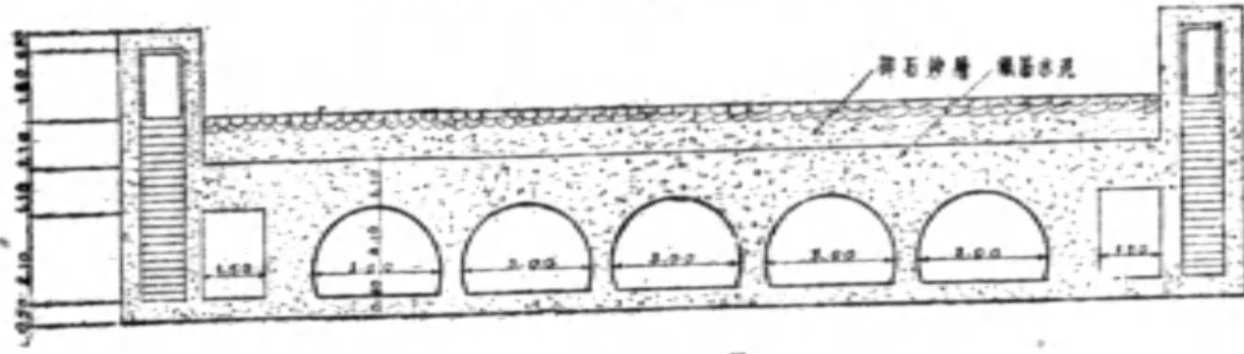
斷面圖
