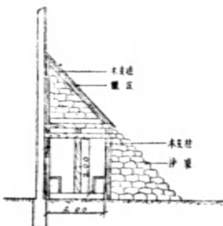
斷面圖
