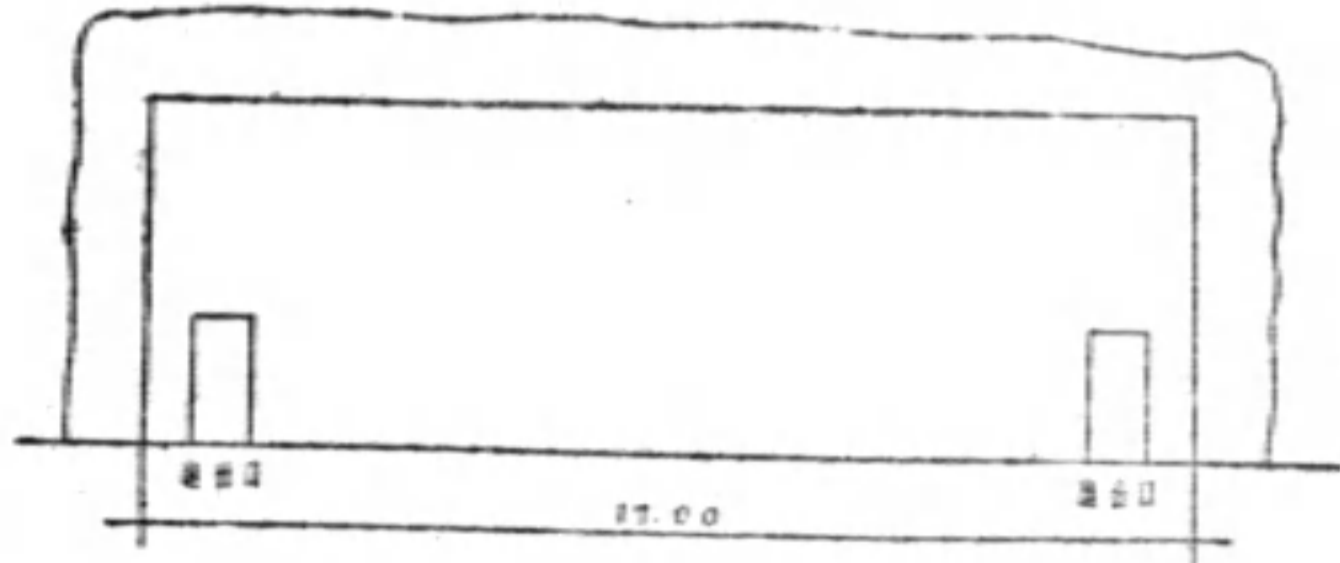
半圓形避難所正面圖 防禦百公斤炸彈可容五十人避難
