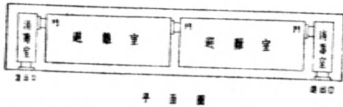
地連射避難所平面圖 防護百公斤炸彈可容六十人避難
