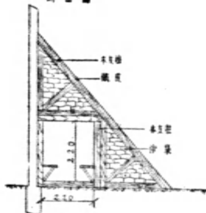
斷面圖
