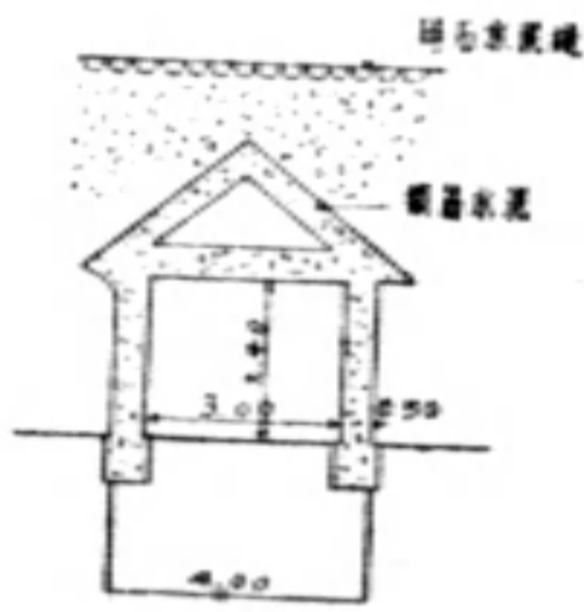
斷面圖
