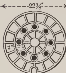
FIG. 7. BROOKLYN, (N. Y.) MANHOLE COVER, 1896. AVE. WEIGHT, HEAD, 395 LBS. " " COVER, 130 "
