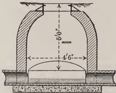
FIG. 2. SHALLOW MANHOLE.
