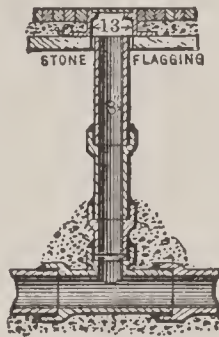
FIG. 10. PIPE LAMPHOLE.
