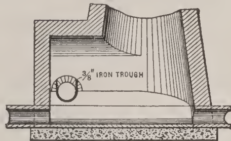
FIG. 3. SHALLOW MANHOLE.
