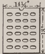
FIG. 2. INLET.
