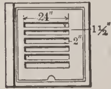
FIG. 2. INLET.
