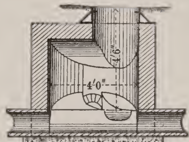
FIG. 3. SHALLOW MANHOLE.
