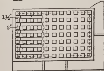
FIG. 9 VENTILATING MANHOLE HEAD.
