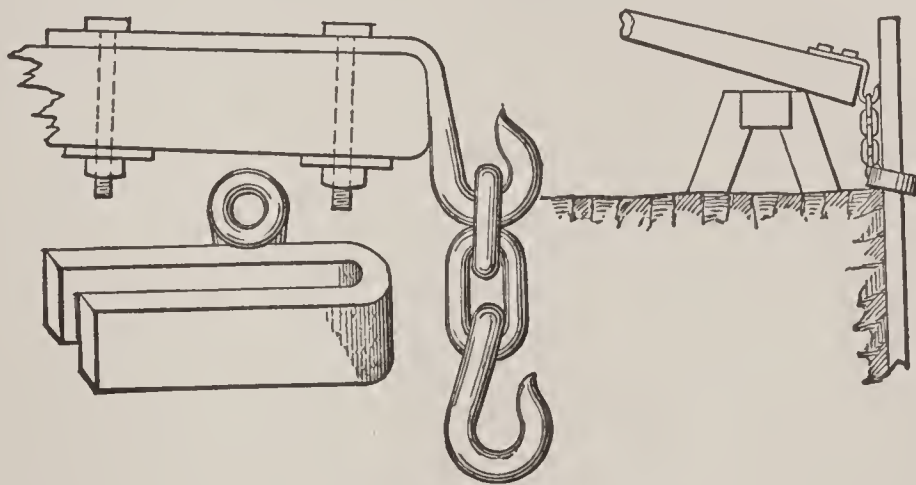
FIG. 18.—SHEATHING-PULLER.
