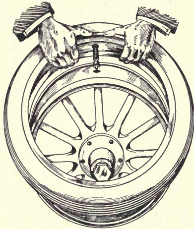
Fig. 134. Returning Tire to Rim.
