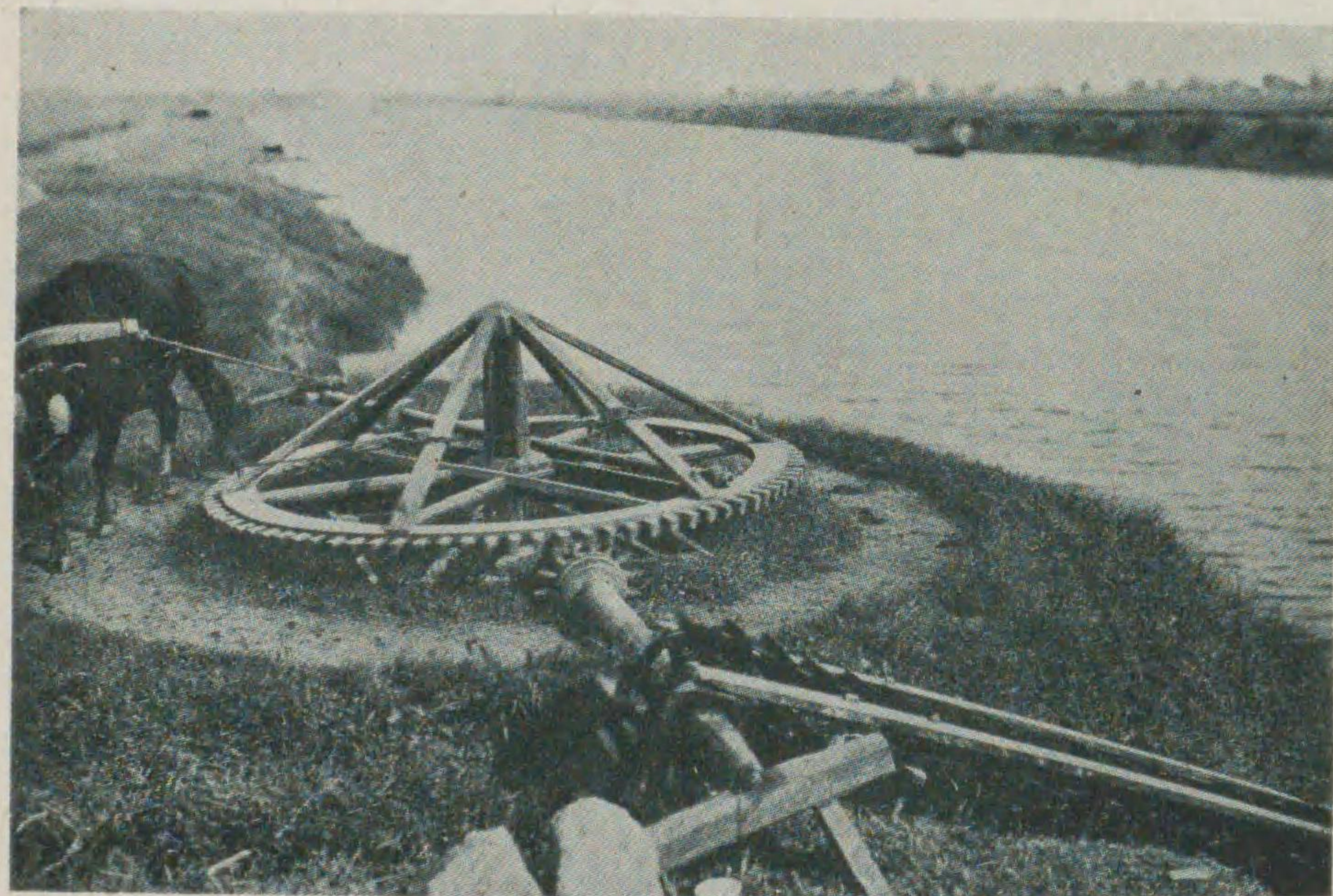
造構の車骨龍る見に方地蘇江、江浙 (四十)
