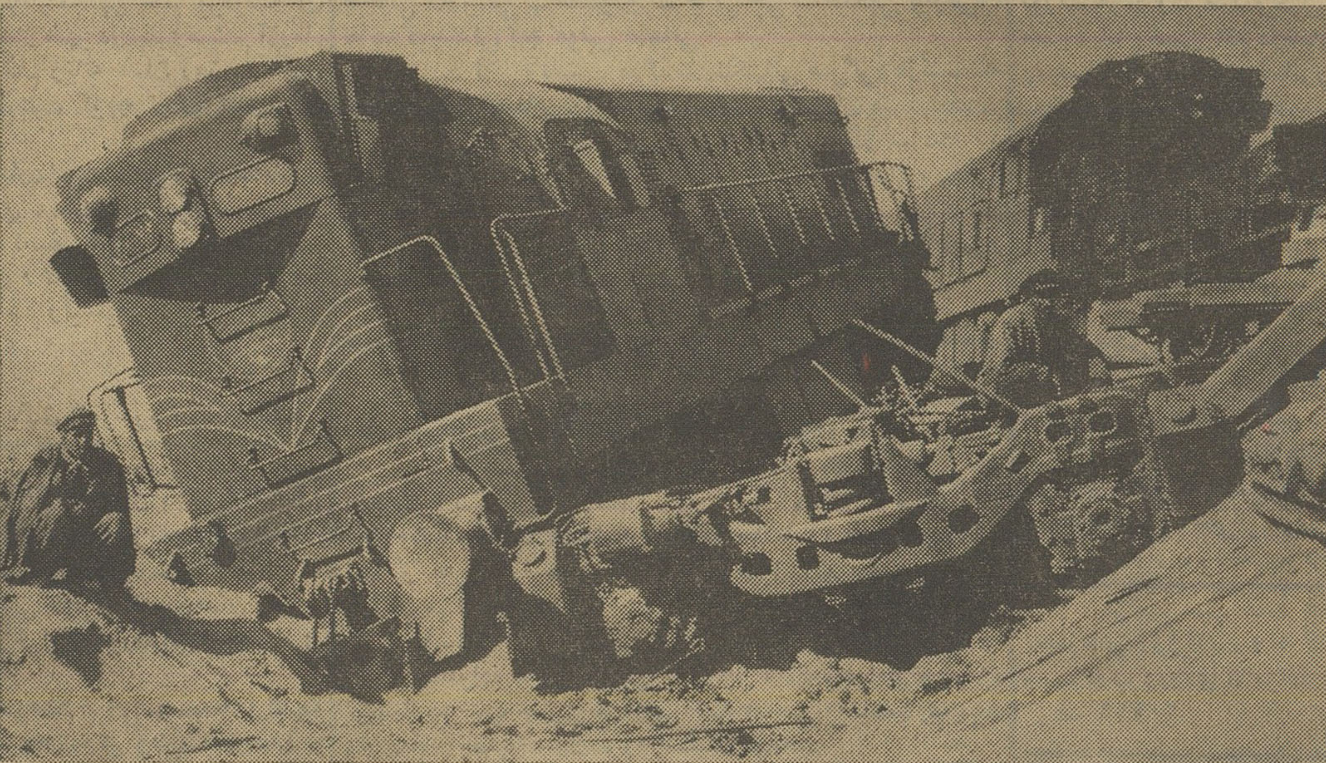
لکوموتیو دیزل که از خط خارج شده است
