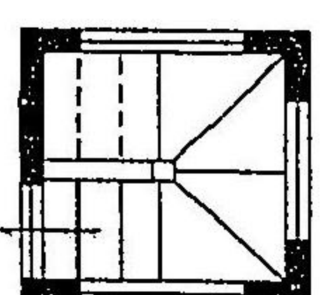
第七十九圖 屋上出口階段
