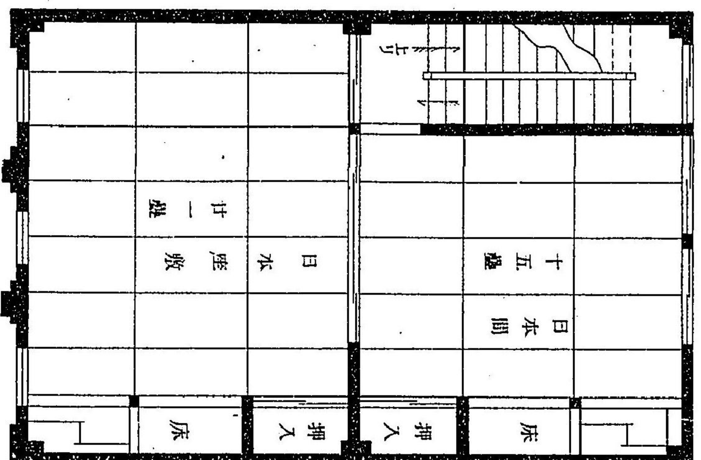
第七十八圖 階下平面
