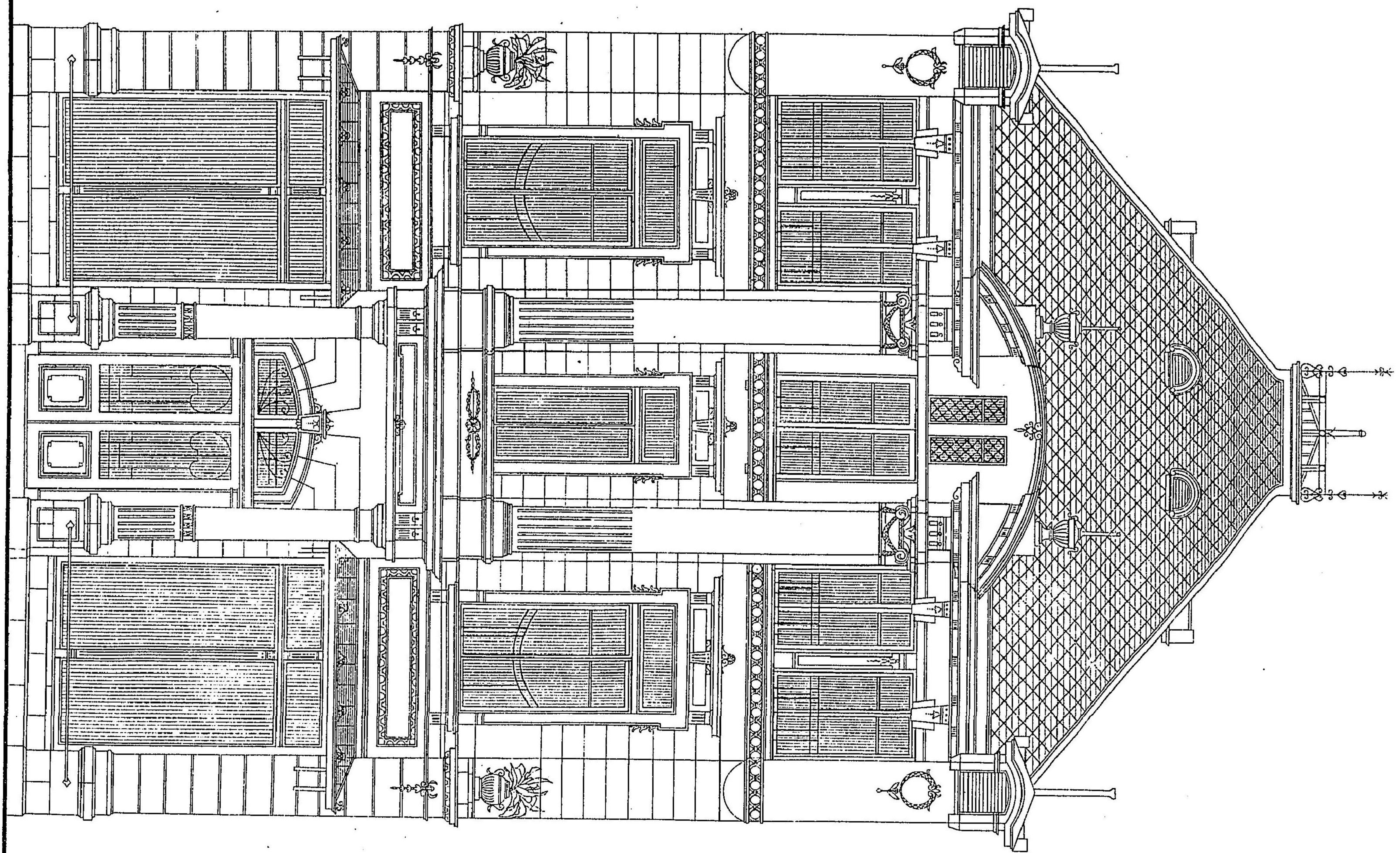
第二十四號商店設計圖 第六十九圖
