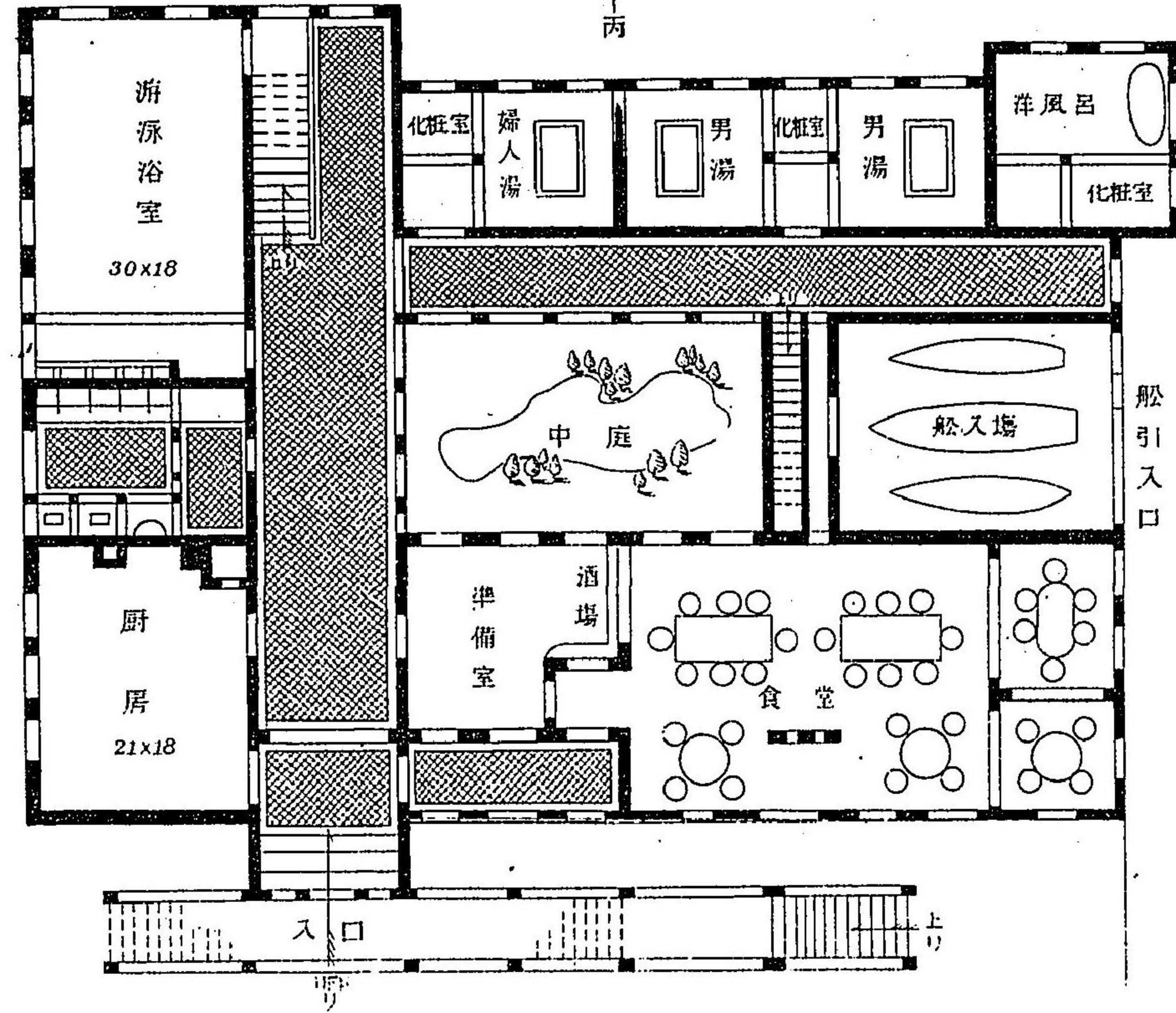
第九十三圖 地階平面
