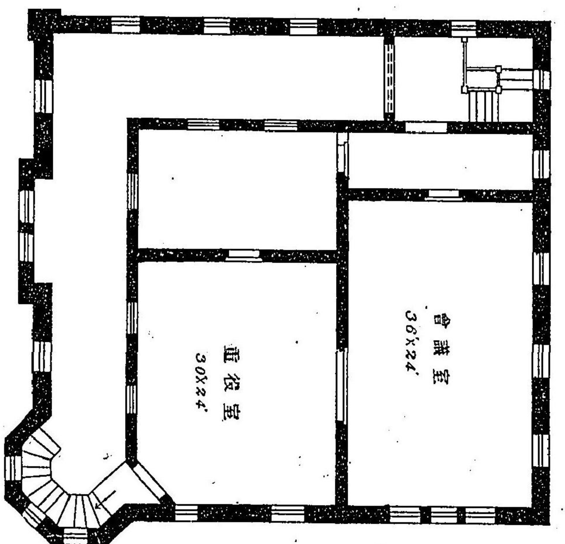
第一百十二圖 階上平面
