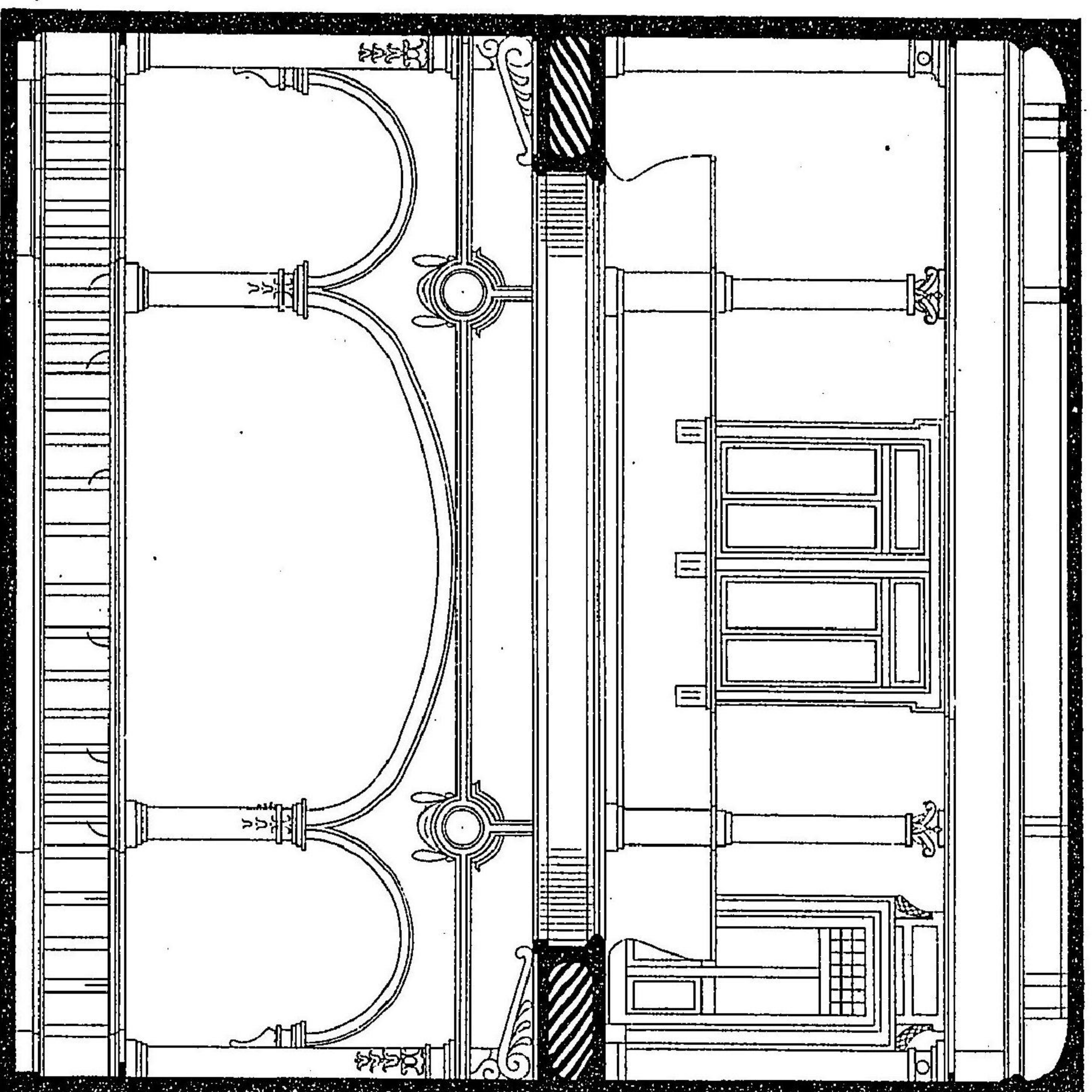
第七十五圖 店橫斷面 尺度五十分之一
