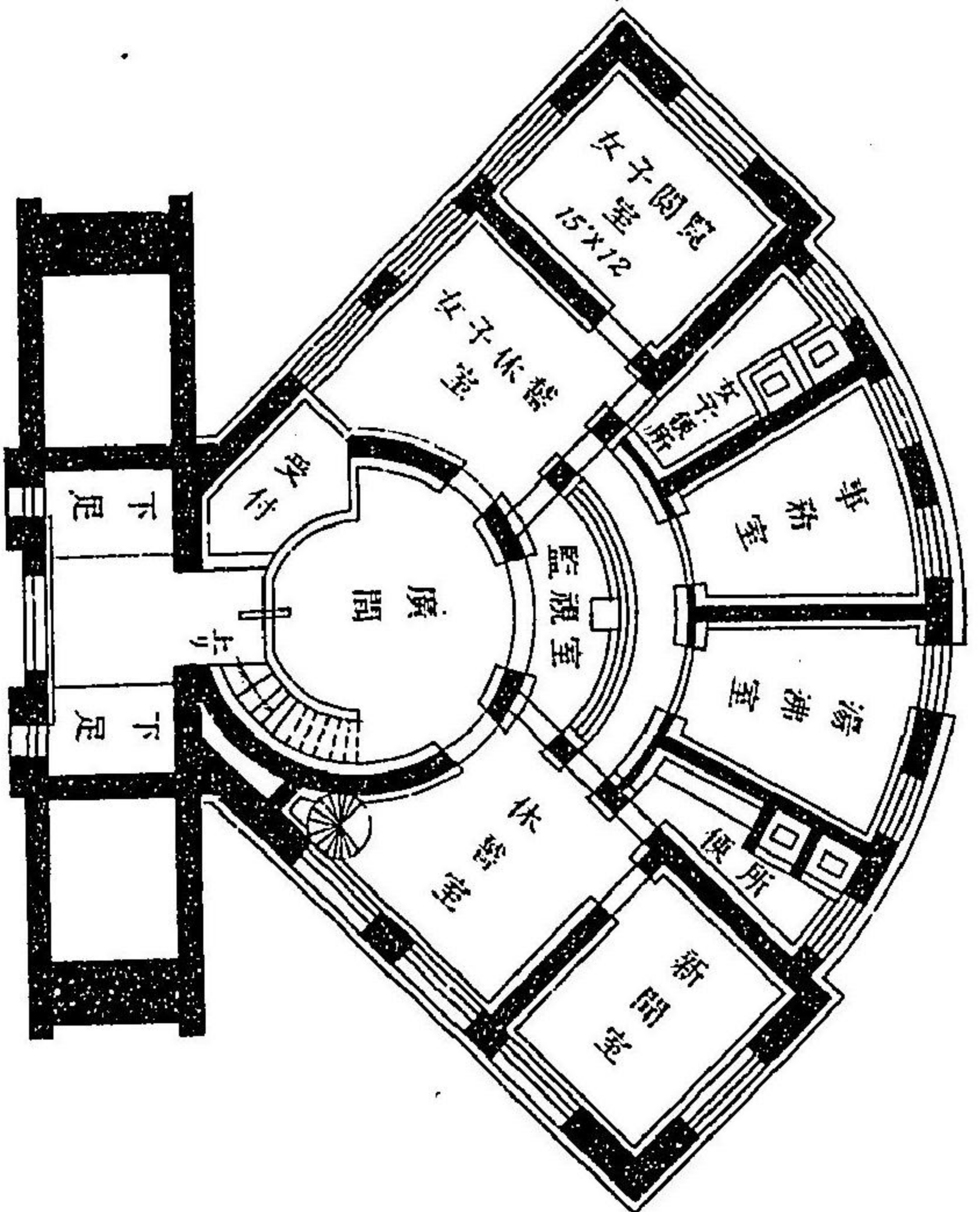
第一百二十一圖
