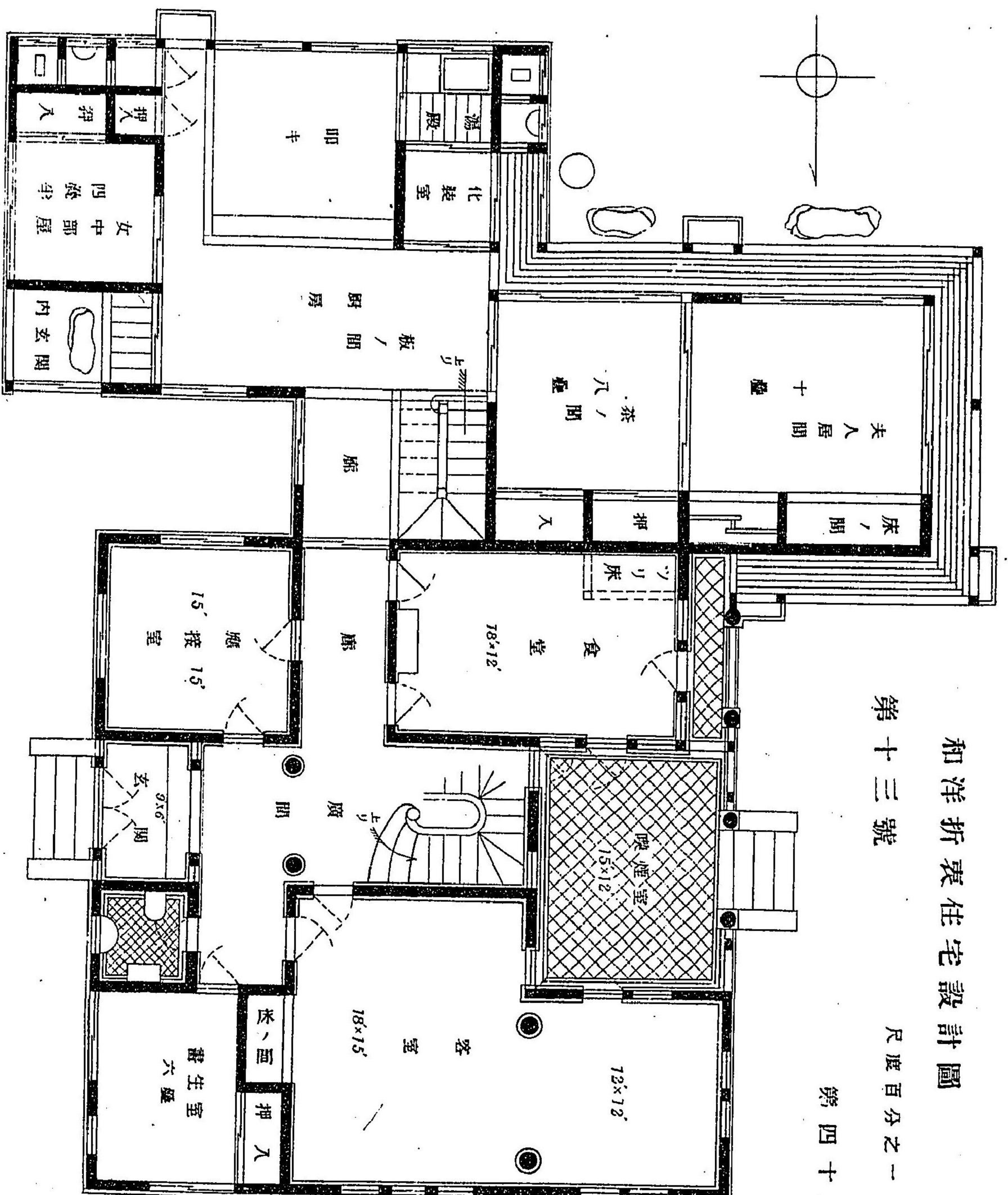
階下平面
