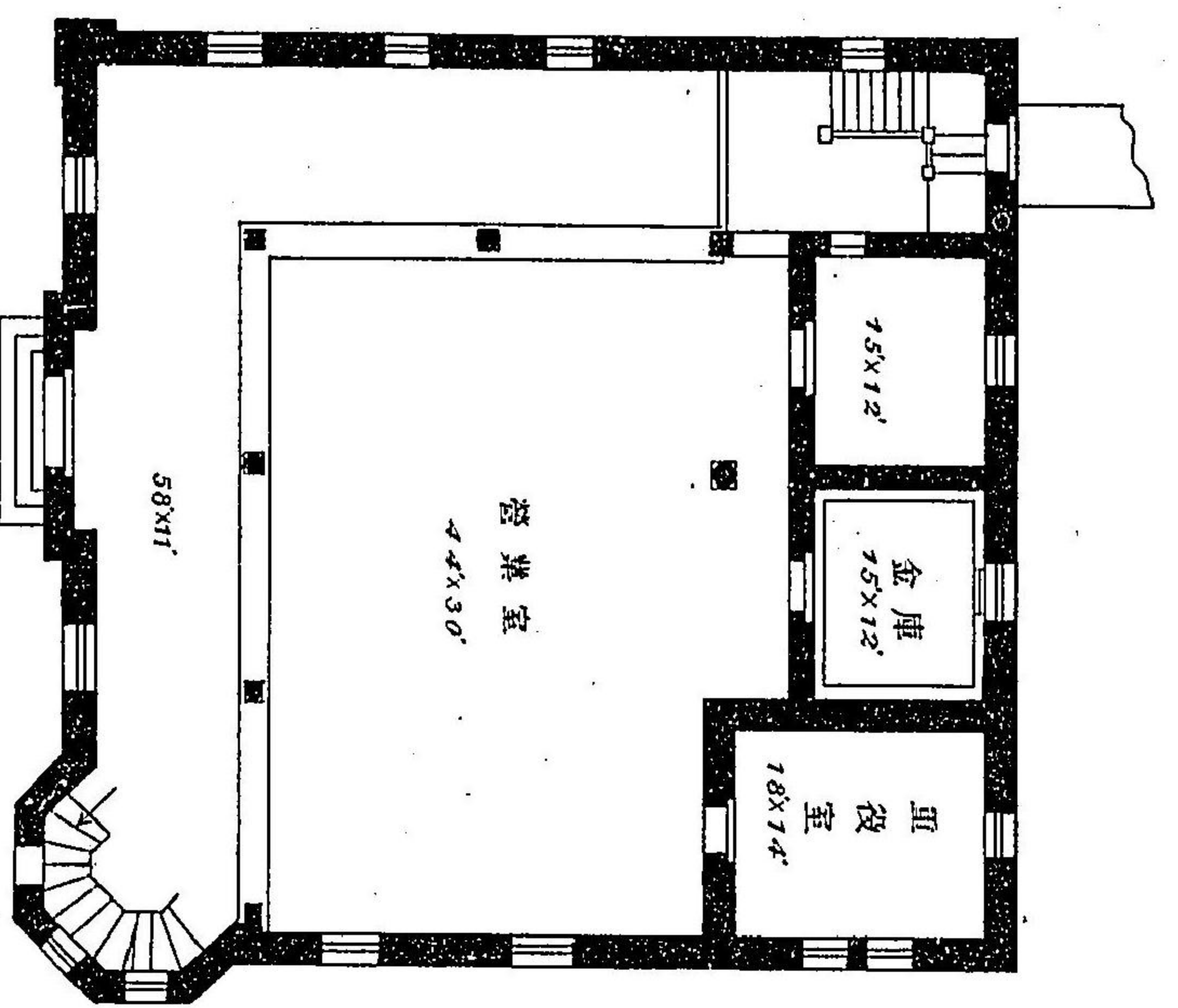
第一百十一圖 階下平面
