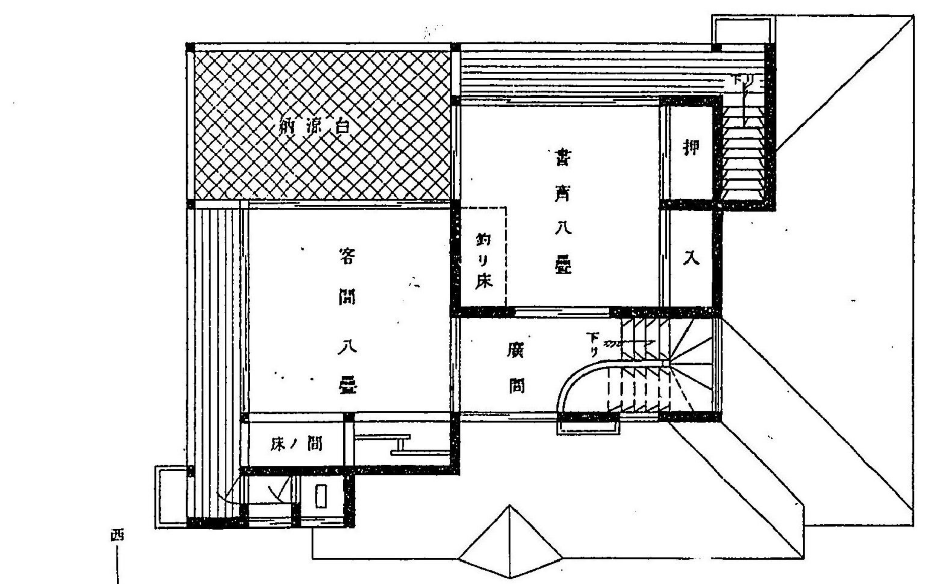
第四號 第九圖
