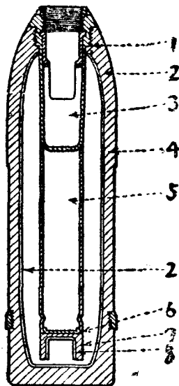
第六十三圖 75 毫米催淚砲彈
