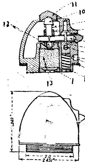
第四十七圖 M—XI 式化學迫擊砲彈引信
