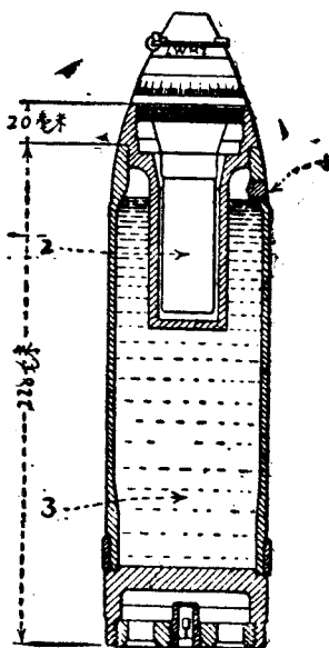
第七十圖 7.7 厘米迫擊砲毒氣彈（最後形式的D式迫擊砲彈）
