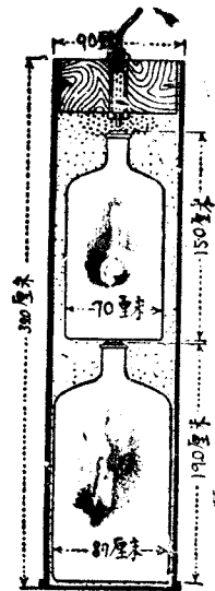
第五十七圖 裝填溴素與 9 厘米迫擊砲彈 (最初形式)
