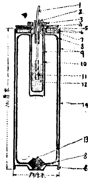
第五十八圖 9 厘米毒氣迫擊砲彈
