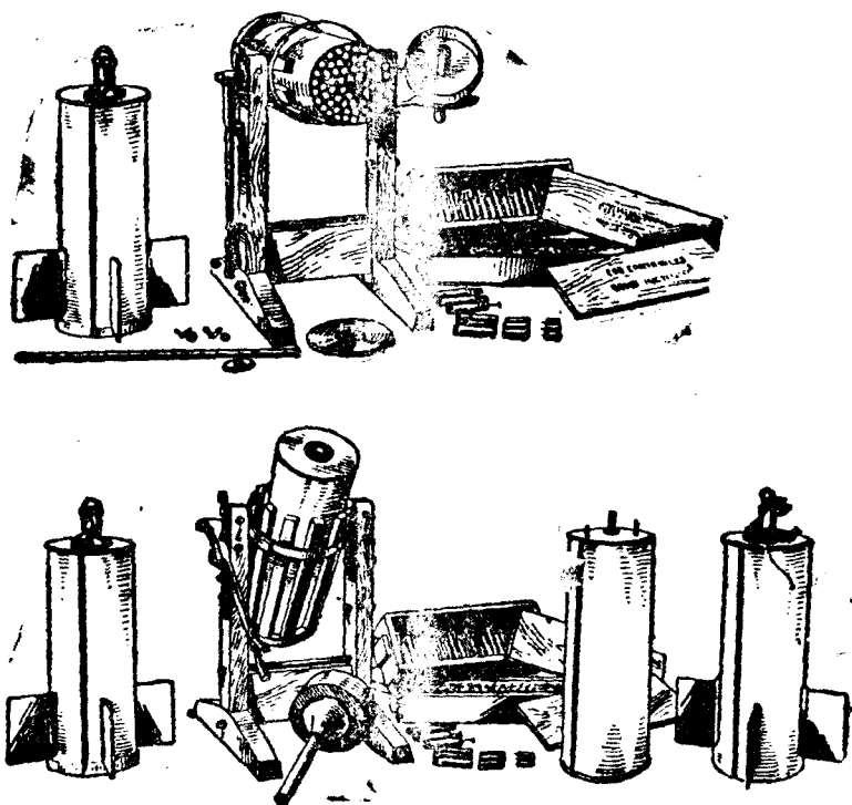
第九十八圖 英國雛形飛機縱火彈
