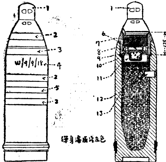
第七十九圖 十八磅砲芥氣砲彈
