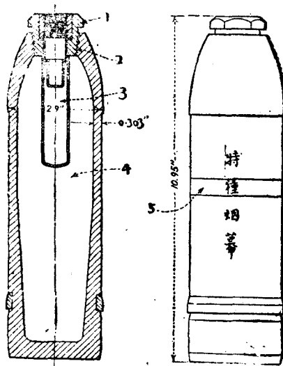
第八十圖 美國 75 毫米化學砲彈
