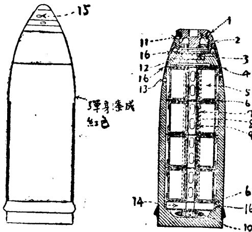
第八十六圖 4.5 英寸縱火榴彈砲彈
