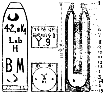
第五十九圖 17 厘米毒氣迫擊砲彈
