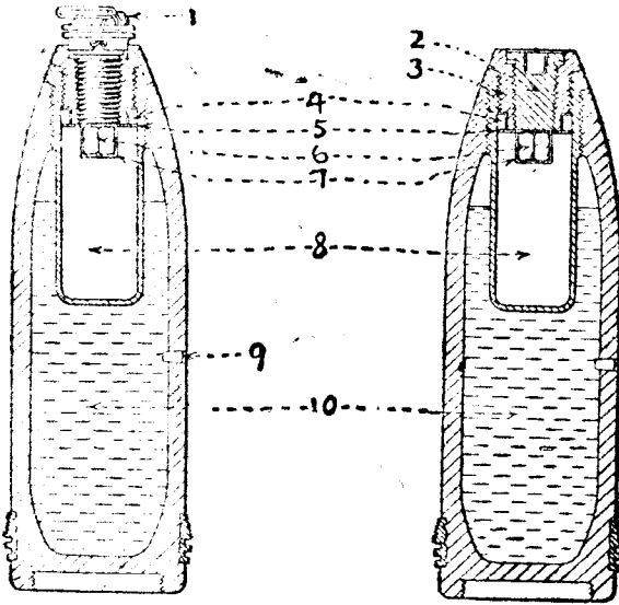
第七十四圖 4.5 英寸榴彈砲毒氣彈 (容器式)
