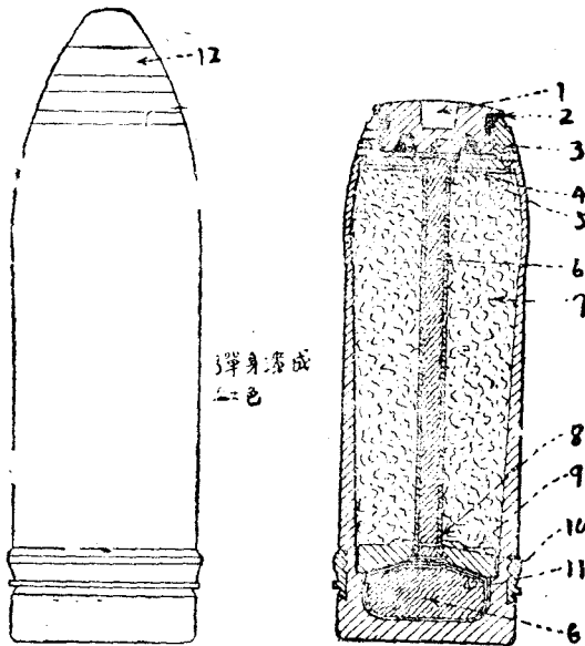
第八十五圖 十八磅砲縱火砲彈
