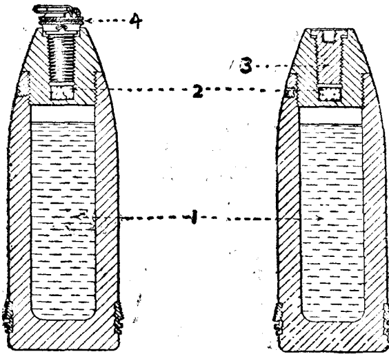
引信裝就的砲彈
