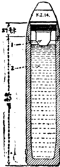
第六十七圖 新式 7.7 厘米毒氣砲彈（長型）
