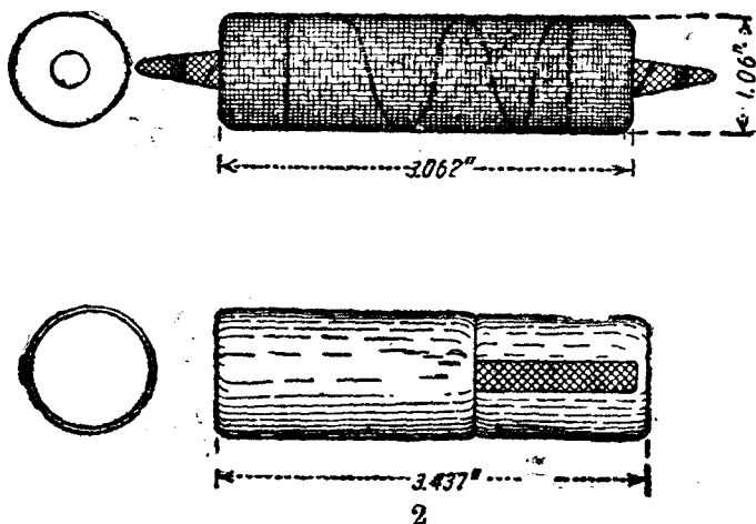
第八十四圖 法國 1878 年式縱火筒
