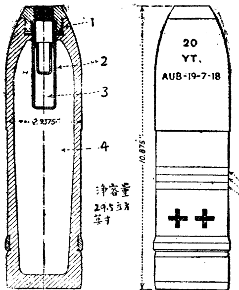
第七十八圖 法國 75 毫米鋼質砲彈 (1915 年式) [國中彈外標識，係表示內含『20 號混合物』(即芥氣)]
