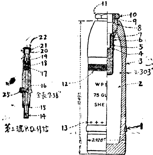
第二號 75 毫米砲彈 (黃磷 彈的專用標記)
