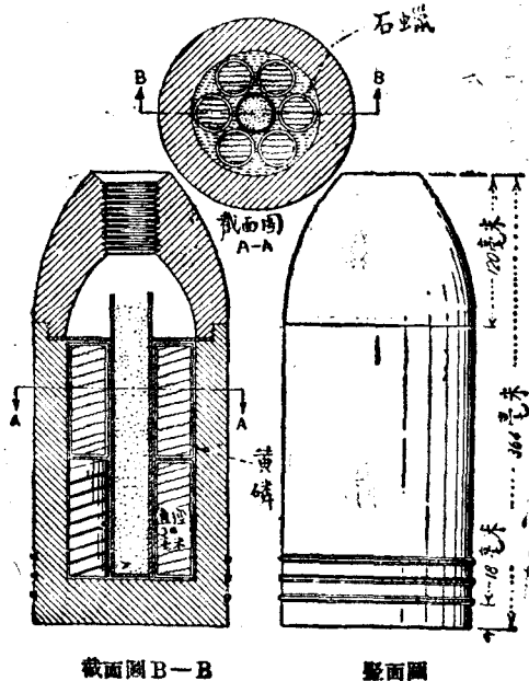
第八十二圖 15 厘米縱火砲彈
