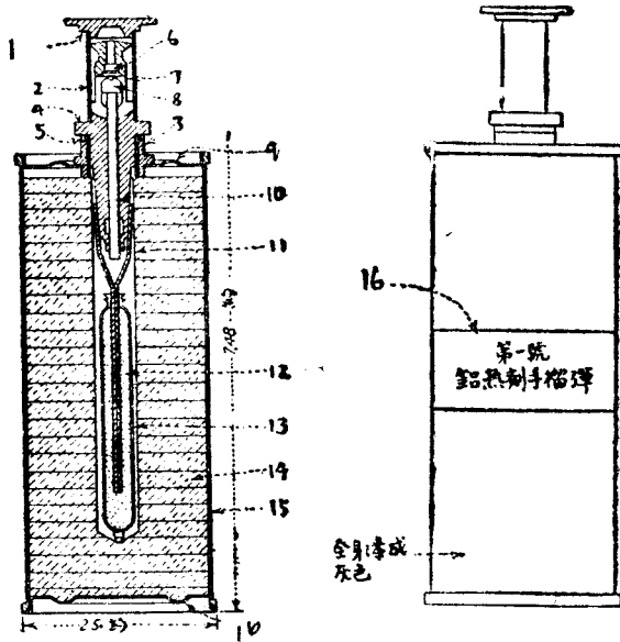
第三十一圖 第一號鋁熱劑手榴彈
