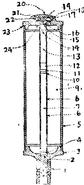
第四十四圖 四英寸托克迫擊砲的毒氣彈
