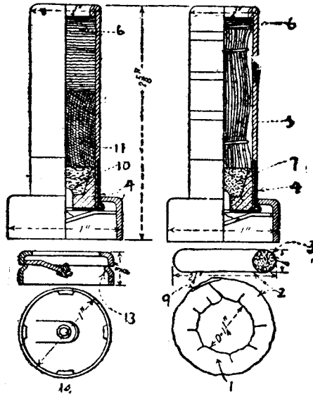
第四十八圖 司托克迫擊砲的發射藥
