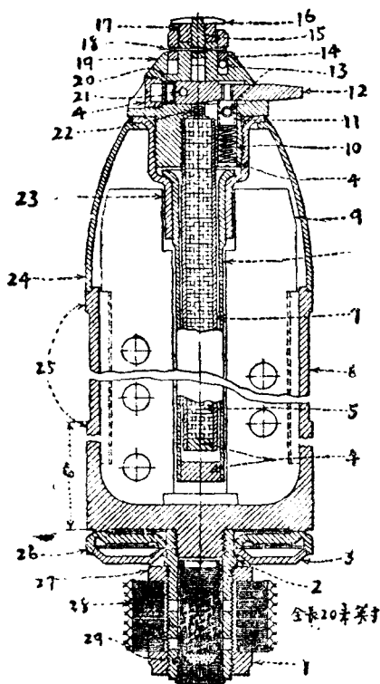
第四十九圖 M-1 式 4.2 英寸化學迫擊砲彈
