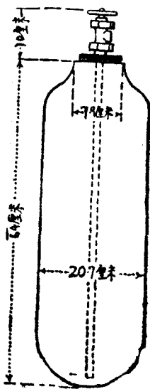
第三十七圖 毒氣吹放瓶 (德國式)
