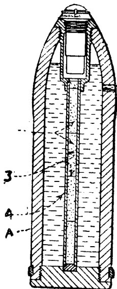
第七十五圖 15 厘米黃十字毒氣砲彈
