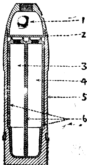
第六十二圖 75 毫米催淚砲彈
