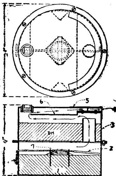
第五十圖 M-I 式 DM 刺激燭
