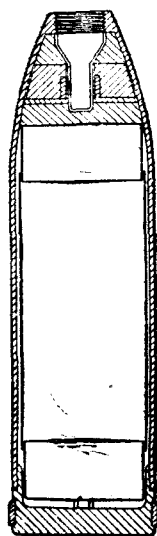
第六十圖 新式 17 厘米毒氣迫擊砲彈*
