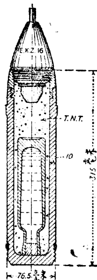
第七十七圖 7.7 厘米藍十字 (噴囊性) 毒氣砲彈
