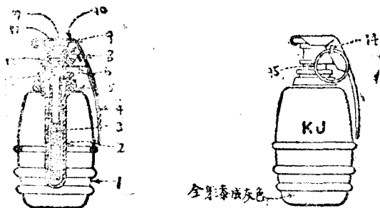
第二十九圖 美國第二號毒氣手榴彈
