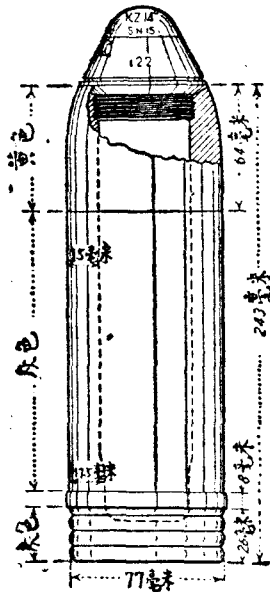
第六十六圖 1915 年式的 7.7 厘米綠十字砲彈
