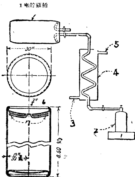
裝填 \text{Cl}_2 或 \text{COCl}_2 的裝置
