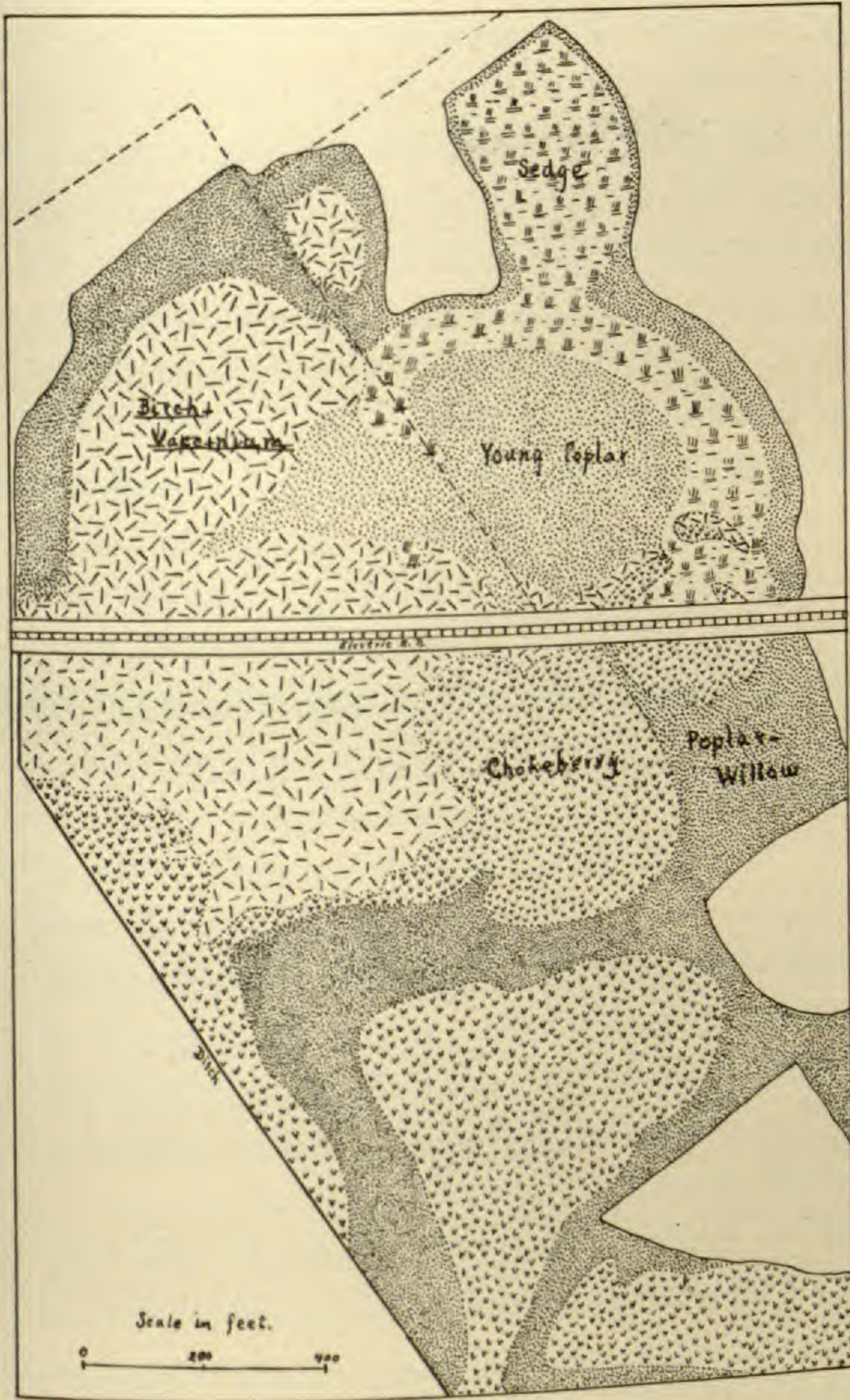
FIG. 11.—Chelsea bog.
