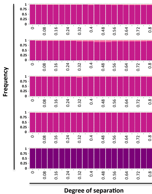
b) \Delta(K)
