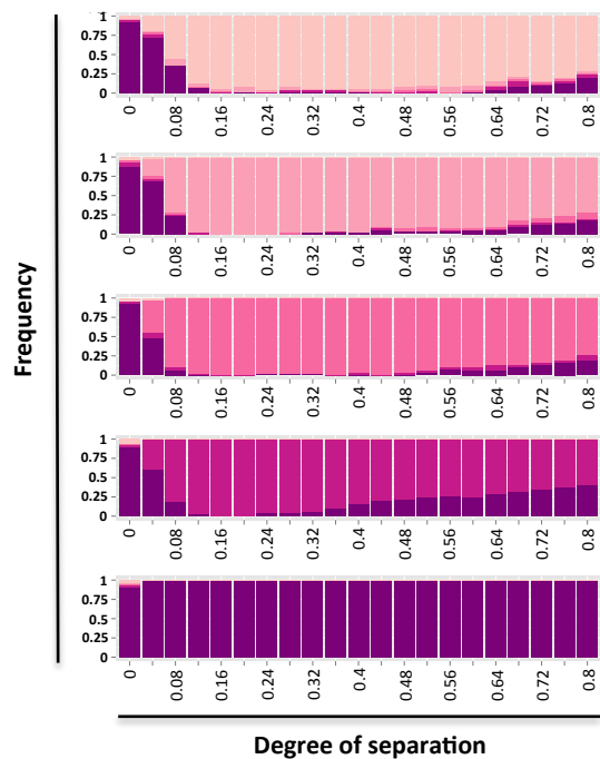
a) PAC
