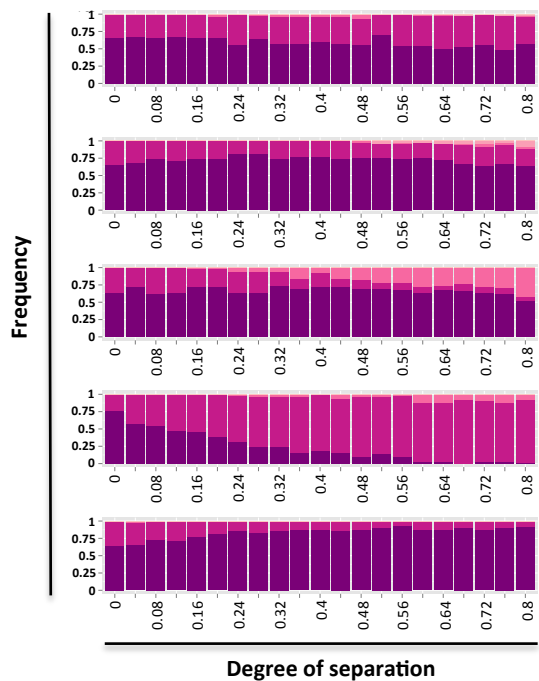
d) GAP-PC
