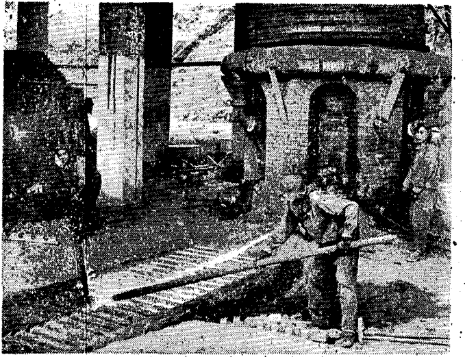
宁乡八一矿厂用电动机带动鼓风，创造高速安全运转3,000小时(150天)的记录。送风风压达1.0兆米水银柱，风量440度，使鼓风效率提高1.3倍。(刘佛成)
