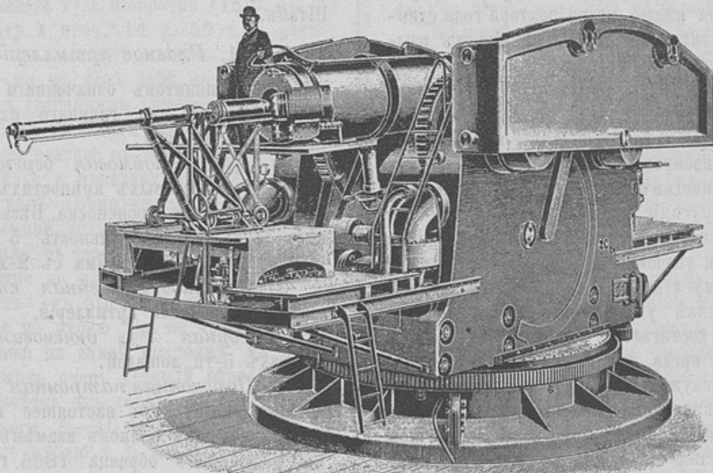
Скрывающійся лафетъ Гордонса, орудіе опущено для заряжанія.
