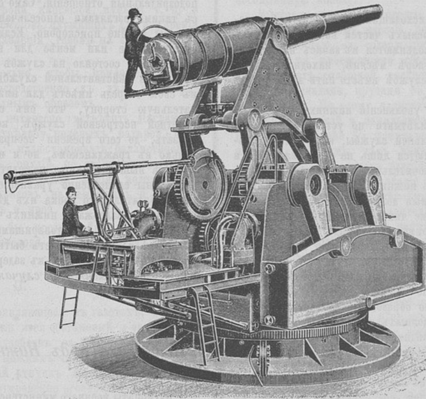
Скрывающійся лафетъ Гордонса, орудіе поднято для выстрѣла.
