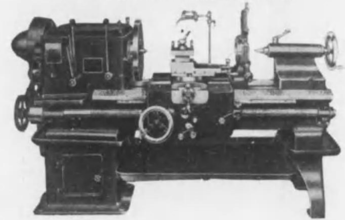
AL型・電動機直結全齒車旋盤
