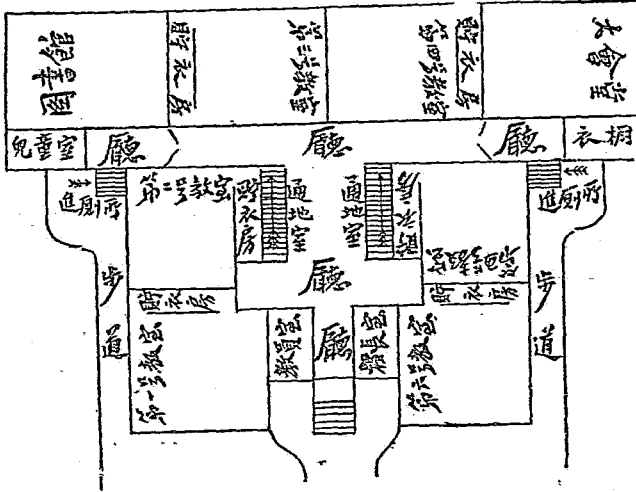
鄉居中樞學校校舍平面圖
