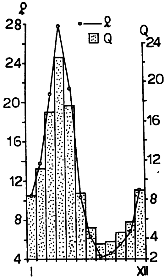
Ск. 3. Графикон протицаја и спец. отицаја код Станичења
