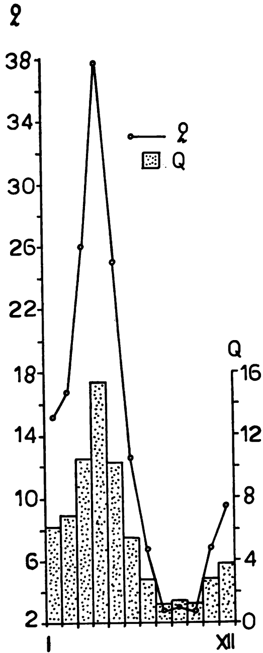
Ск. 1. Графикон протицаја и спец. отицаја код Височке Ржане
