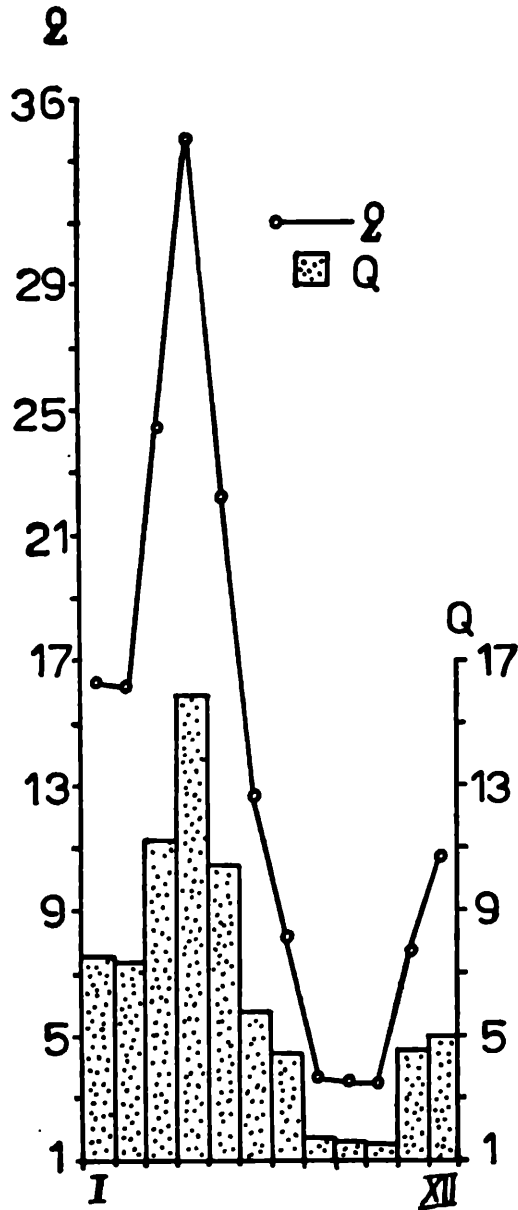
Ск. 2. Графикон протицаја и спец. отицаја код Паклештице
