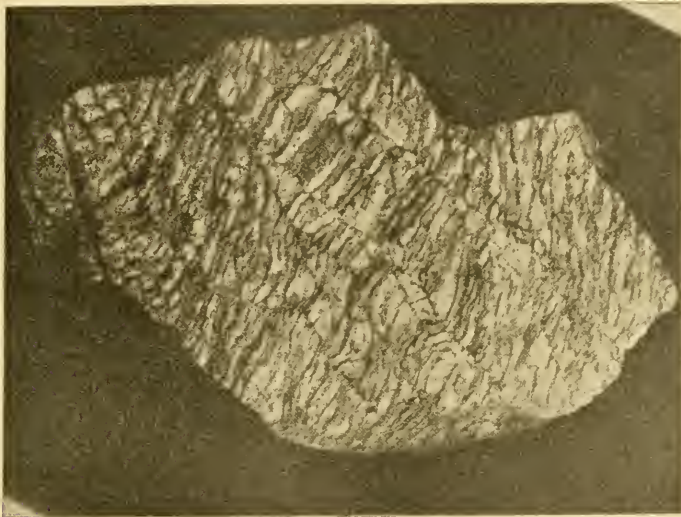
Granit mit scheinbaren Verwerfungen. Dazio grande bei Rodi-Fiesso. \frac{4}{7} d. nat. Gr.
