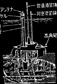
シュノーケル型潜水艦
