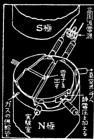
サイクロトロン
