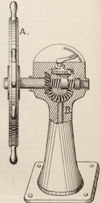
Аксиометръ.
