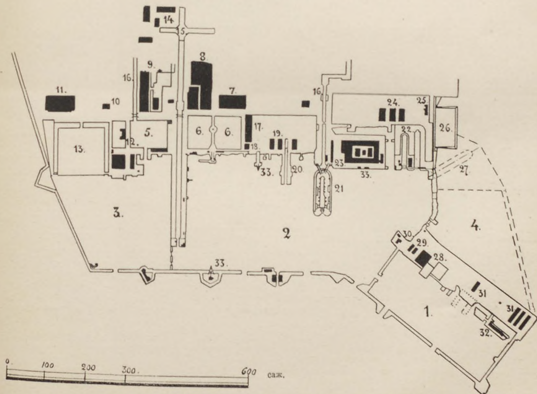
2—Кронштадтскія Адмиралтейства.
